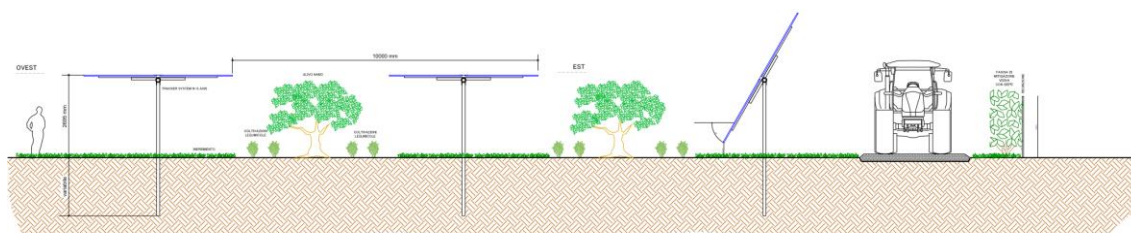
Figura 17 - Sezione tipo impianto
