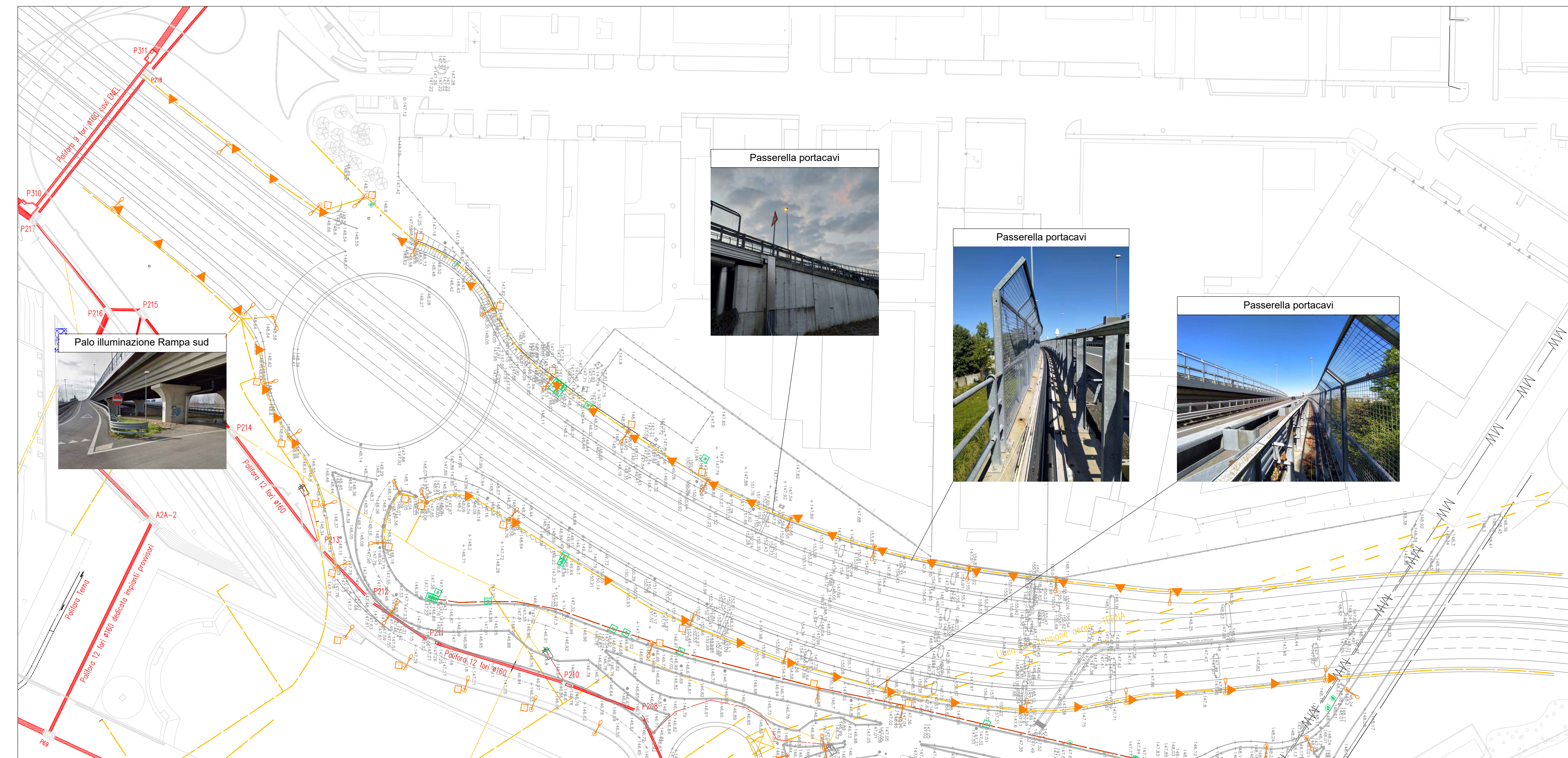
PLANIMETRIA INTERFERENZE POLIFORE - scala 1:1000
