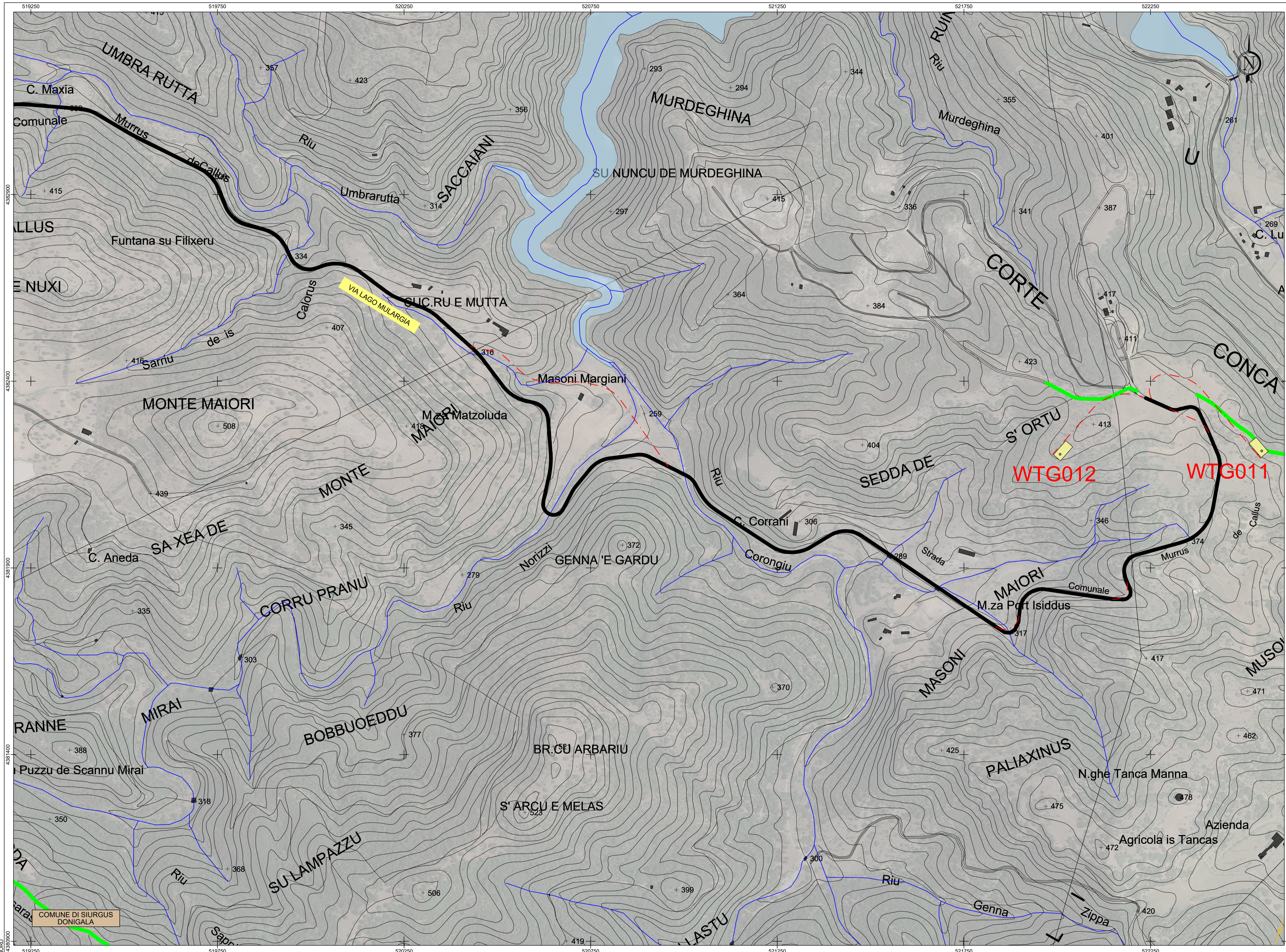
PLANIMETRIA STATO DI FATTO: TAVOLA H Base carta: Carta Tecnica Regionale 1:10.000 e Ortofoto Google Map
