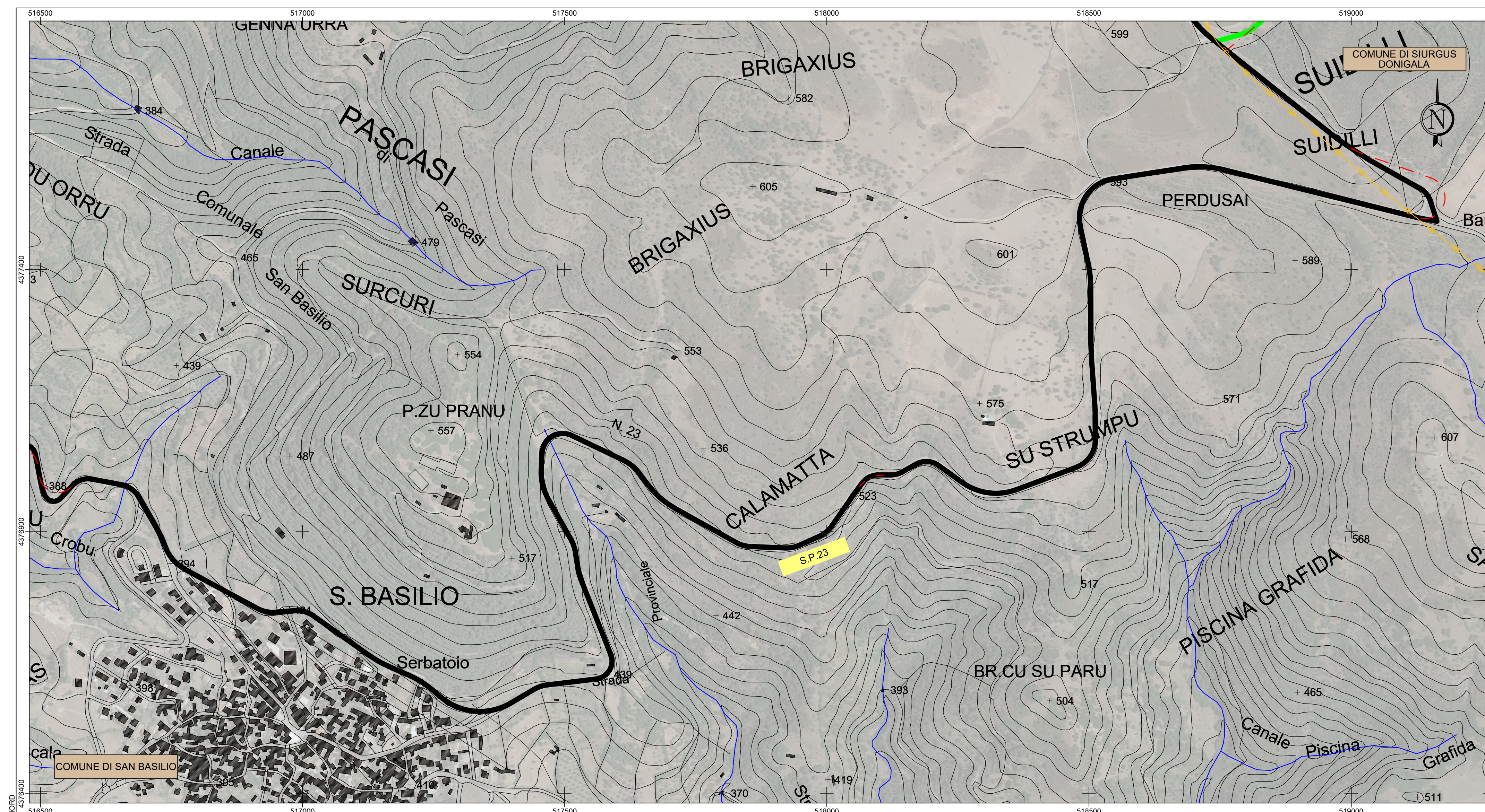
PLANIMETRIA STATO DI FATTO: TAVOLA D.2 Base carta: Carta Tecnica Regionale 1:10.000 e Ortofoto Google Map
