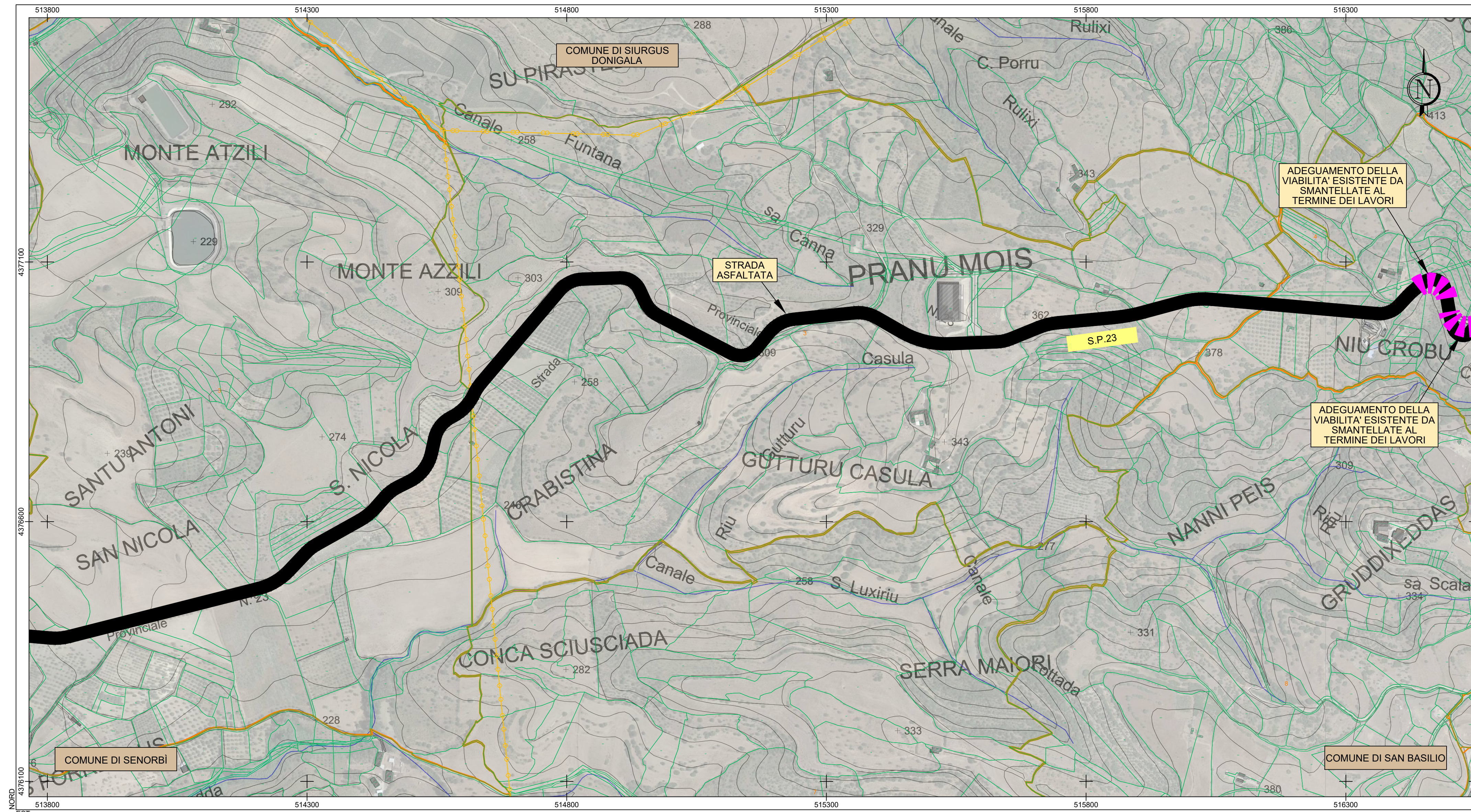
PLANIMETRIA DI PROGETTO: TAVOLA D.1 Base carta: Carta Tecnica Regionale 1:10.000 e Ortofoto Google Map
