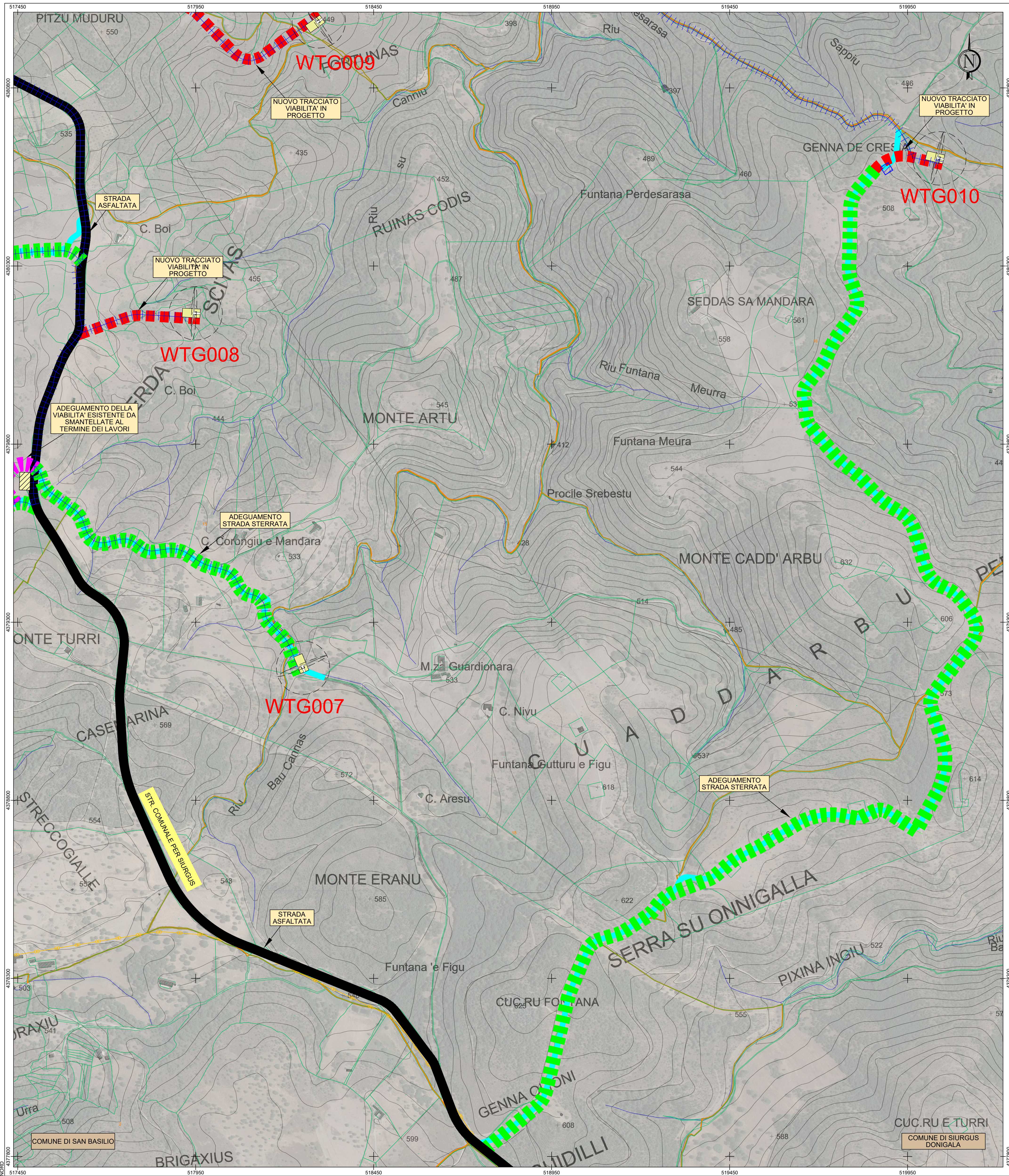
PLANIMETRIA DI PROGETTO: TAVOLA E Base carta: Carta Tecnica Regionale 1:10.000 e Ortofoto Google Map
