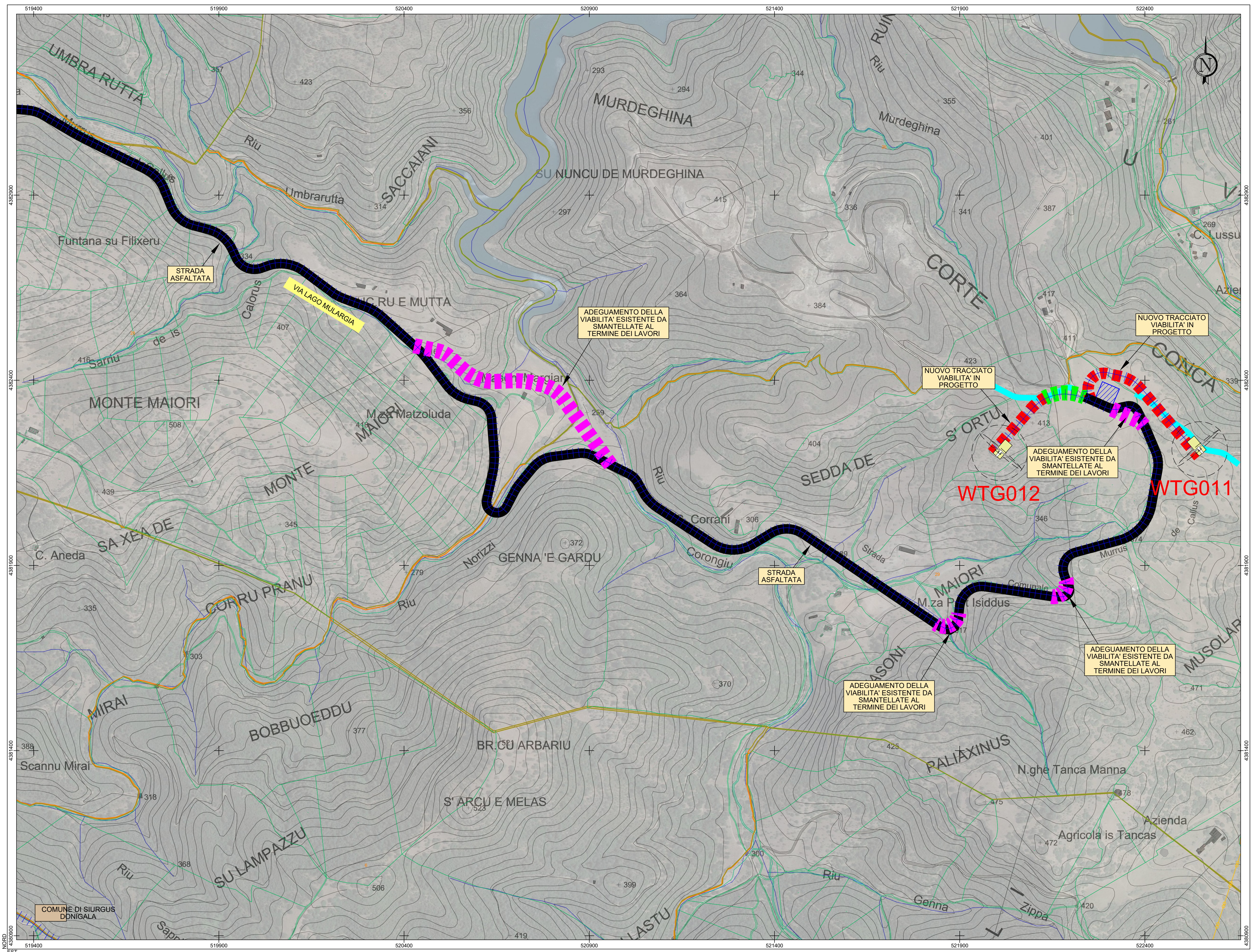
PLANIMETRIA DI PROGETTO: TAVOLA H Base carta: Carta Tecnica Regionale 1:10.000 e Ortofoto Google Map
