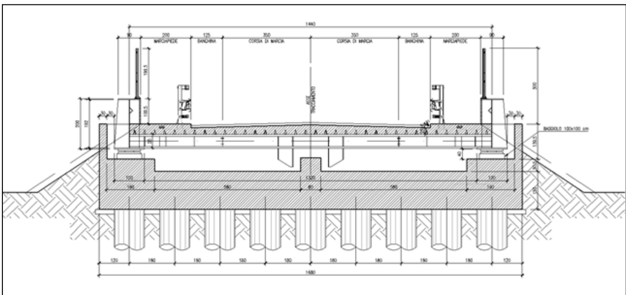
FIGURA 3.1.4 – PARTICOLARE SEZIONE STRADALE CON EVIDENZA OPERE STRUTTURALI E FONDAZIONE
