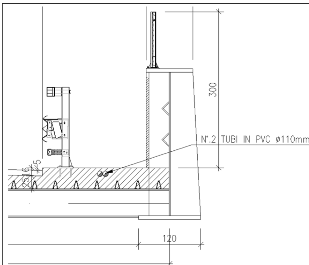
FIGURA 3.2.3 – PARTICOLARE TUBAZIONI DI RACCOLTA SOTTO MARCIAPIEDE
