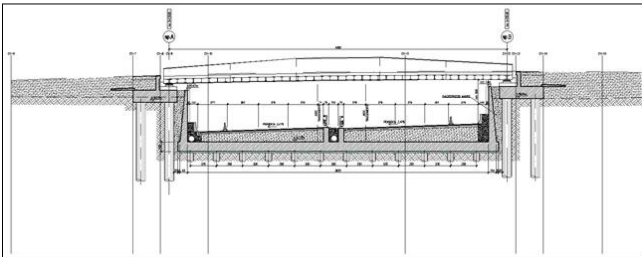
FIGURA 3.1.4 – PARTICOLARE SEZIONE AUTOSTRADALE CHE EVIDENZIA LO SVILUPPO LONGITUDINALE DEL CAVALCAVIA
