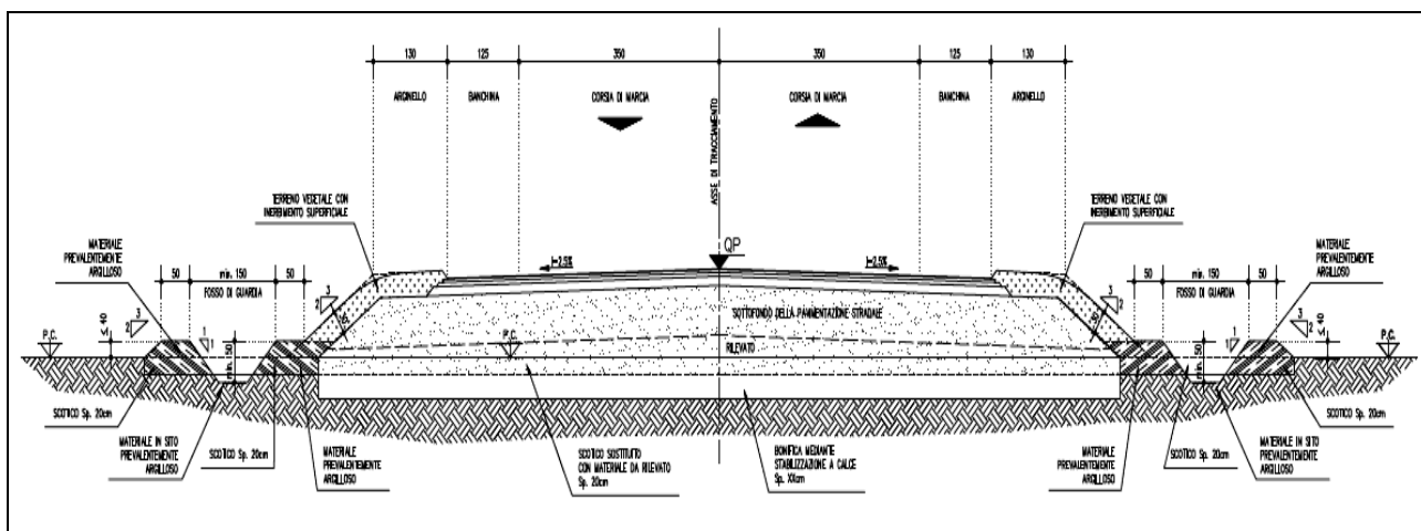
FIGURA 3.1.1 – DEFINIZIONE ILLUSTRATIVA DEGLI ELEMENTI COMPONENTI LO SPAZIO STRADALE
