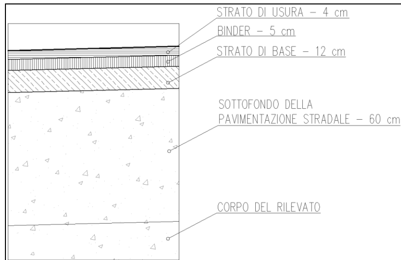
FIGURA 3.1.3 – PARTICOLARE PACCHETTO STRADALE
