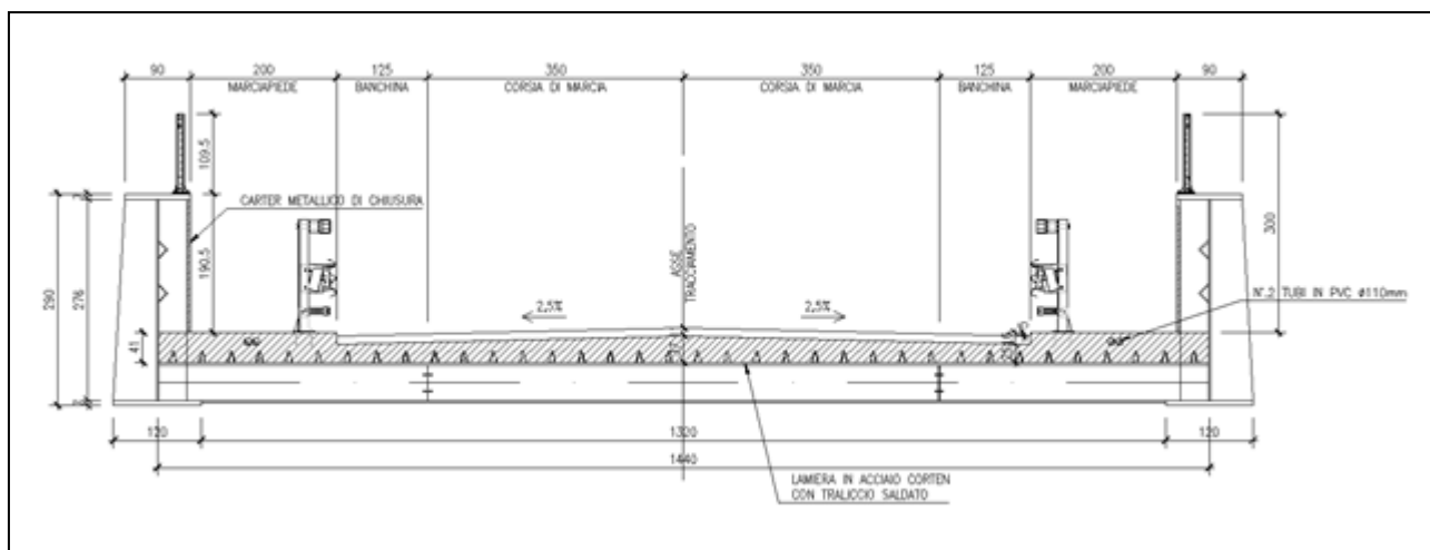
FIGURA 3.1.2 – SEZIONE TIPO STRADA STATALE DELL'ABETONE SUL CAVALCAVIA IN PROGETTO
