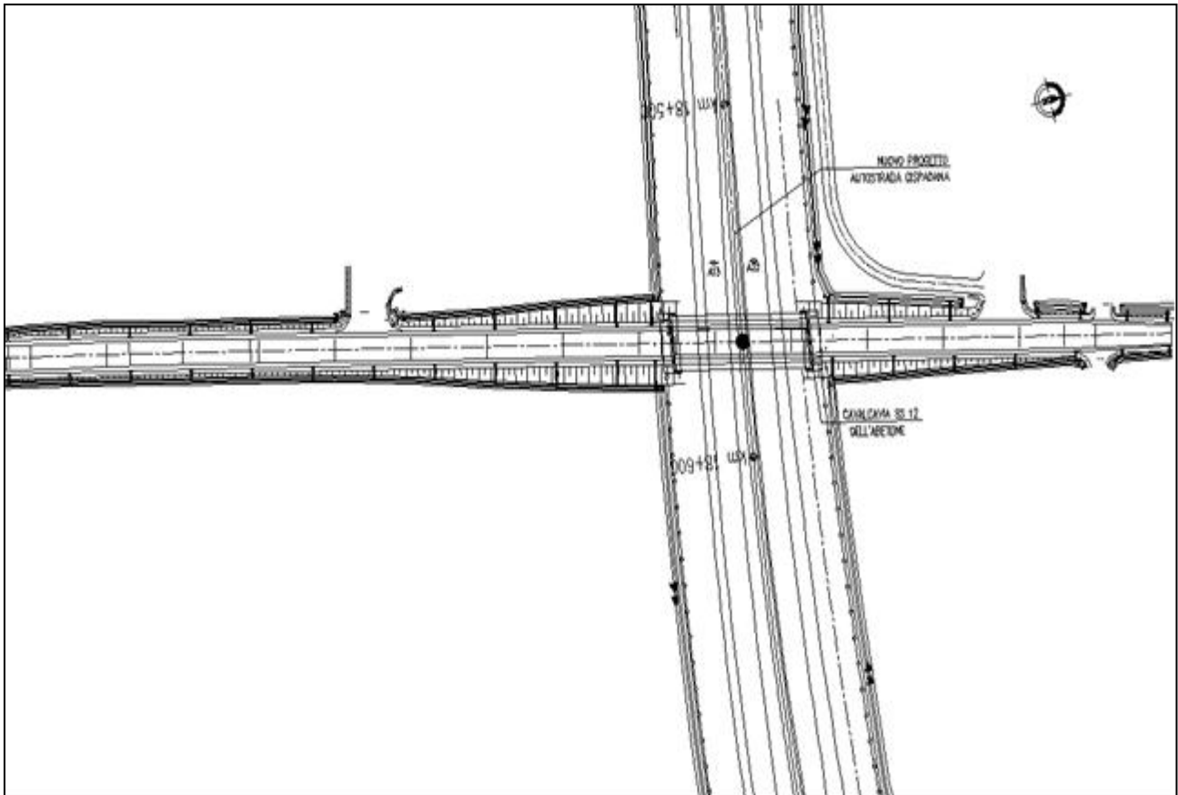
FIGURA 1.1 – SCHEMA PLANIMETRICO DELLA INTERFERENZA TRA AUTOSTRADA E SS12 DELL'ABETONE
