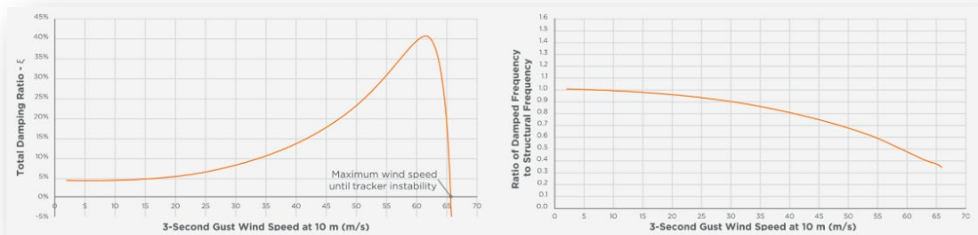
Figura 5 a sinistra FAM: rapporto di smorzamento/velocità del vento - a destra: rapporto di frequenza/velocità del vento
