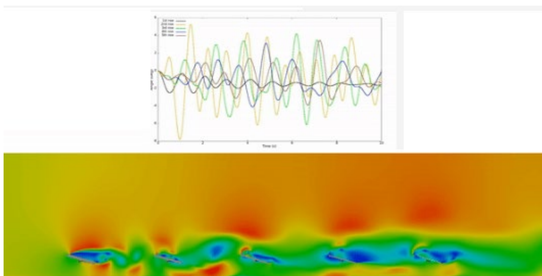
Figura 3 Simulazioni CFD eseguite da Soltec in collaborazione con Lynx basate sulla metodologia Dy-Wind
