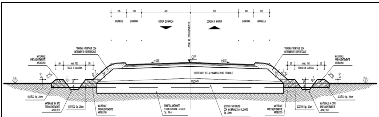
FIGURA 3.1.2 – SEZIONE TIPO STRADA COMUNALE S.ANTONIO DI NUOVA PROGETTAZIONE
