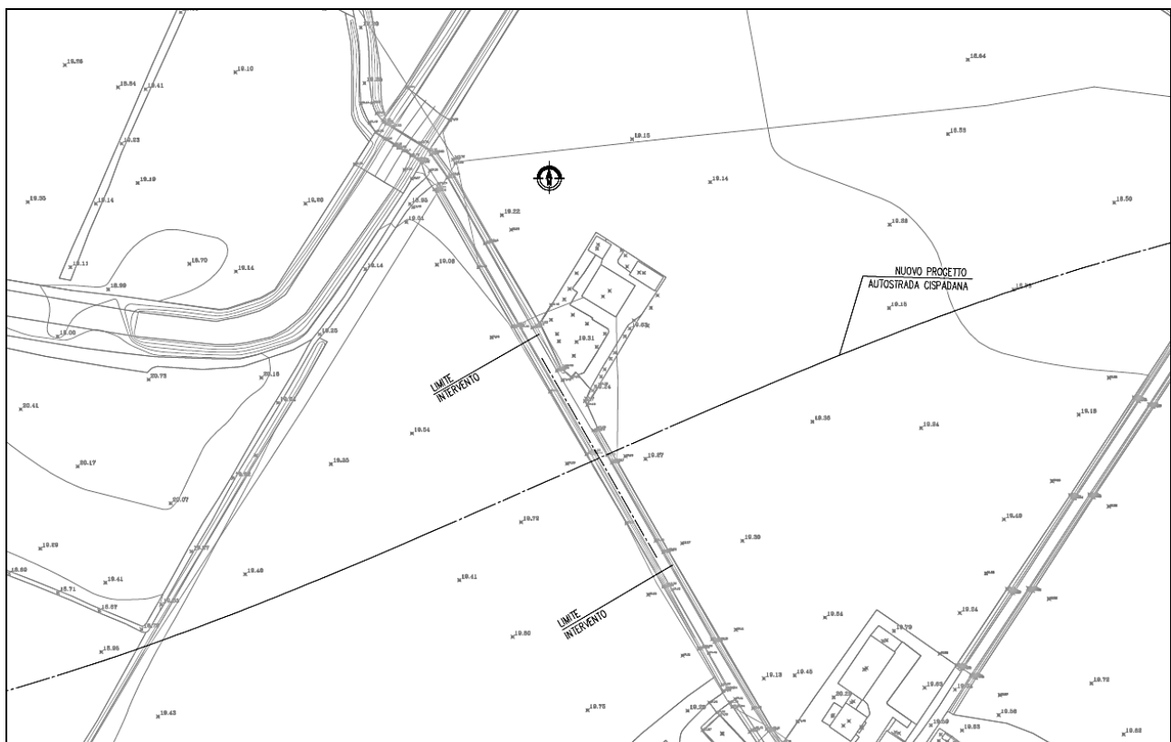
FIGURA 4.1 – STRADA COMUNALE S.ANTONIO ALLO STATO DI FATTO
