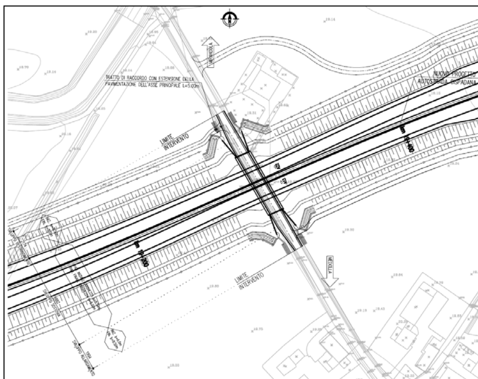
FIGURA 1.1 – SCHEMA PLANIMETRICO DELLA INTERFERENZA TRA AUTOSTRADA E SC S.ANTONIO
