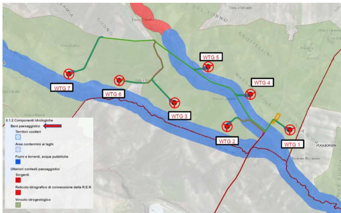
Figura 4 - layout di impianto con le componenti idrogeologiche
