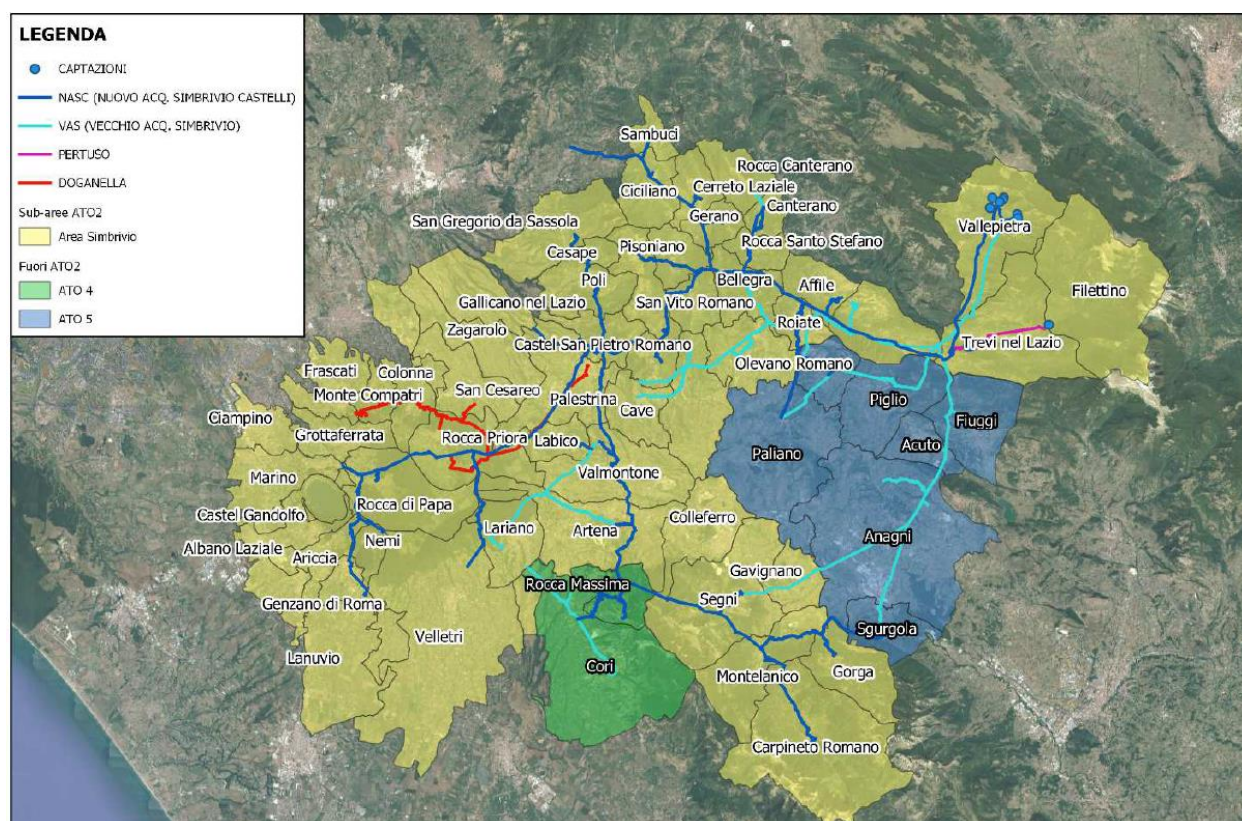
Figura 3-1 Schema di alimentazione dell'Area Simbrivio
