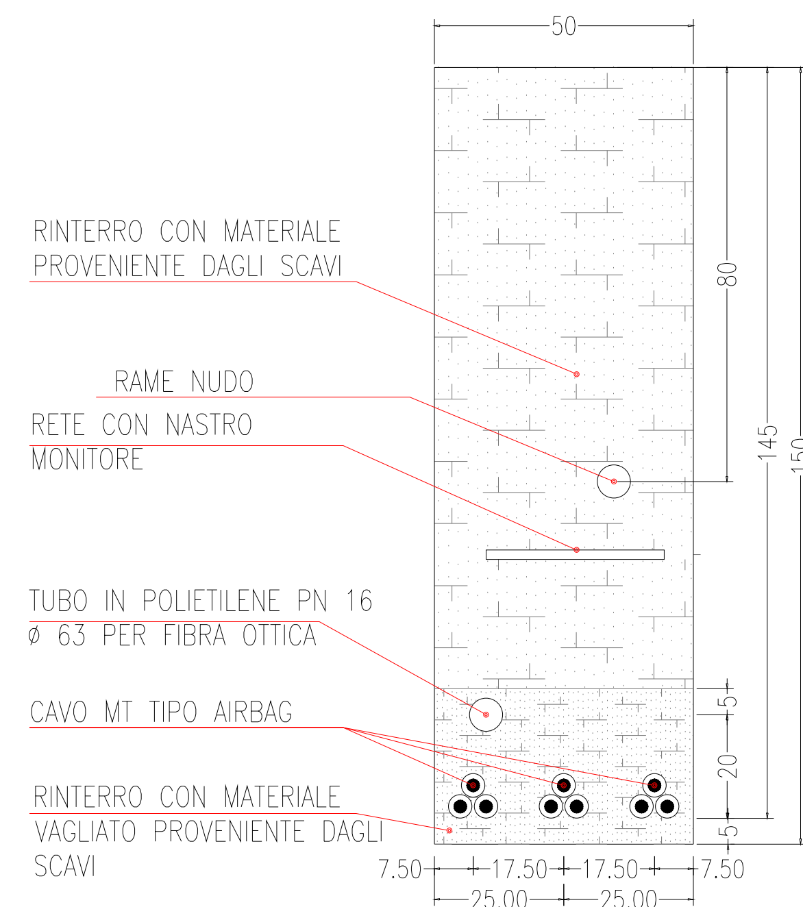
SEZIONE TIPICA C3 SU TERRENO AGRICOLO O TERRENO ALBERATO
