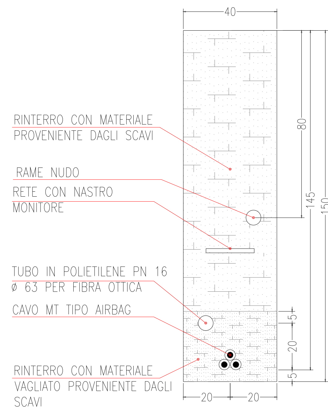
SEZIONE TIPICA C1 SU TERRENO AGRICOLO O TERRENO ALBERATO
