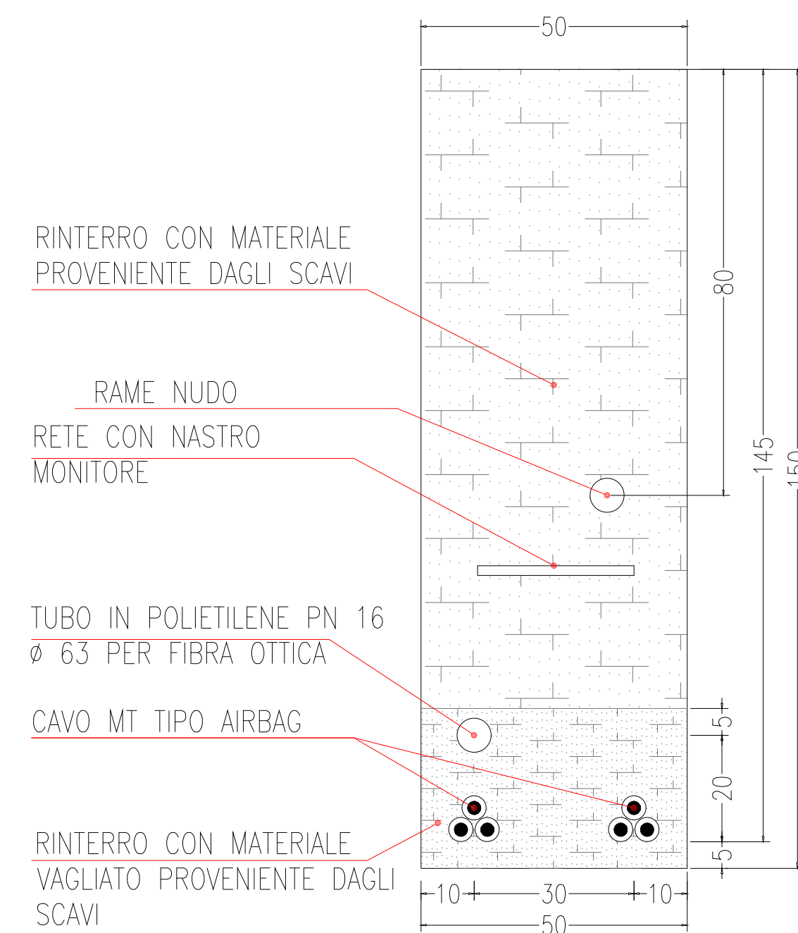
SEZIONE TIPICA C2 SU TERRENO AGRICOLO O TERRENO ALBERATO
