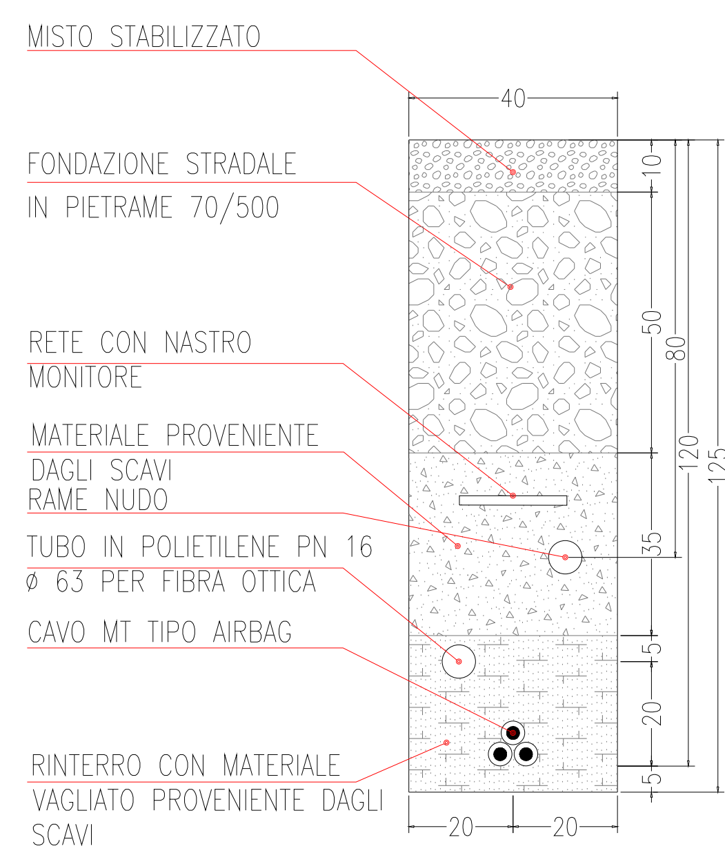
SEZIONE TIPICA C1 SU STRADA NON ASFALTATA
