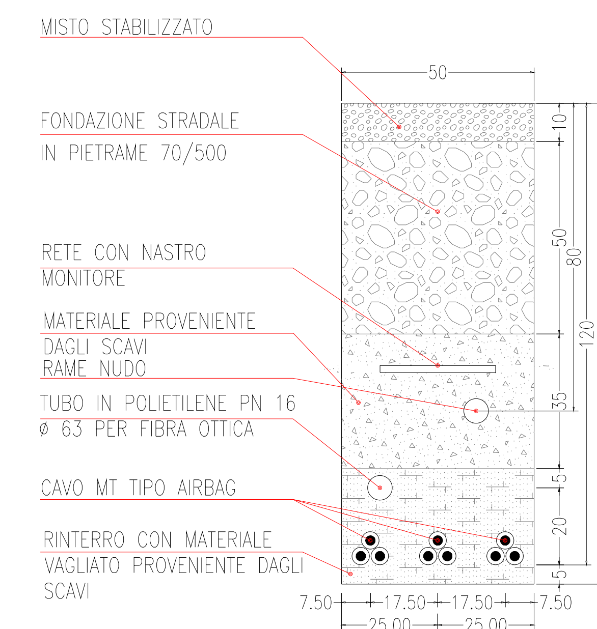
SEZIONE TIPICA C3 SU STRADA NON ASFALTATA
