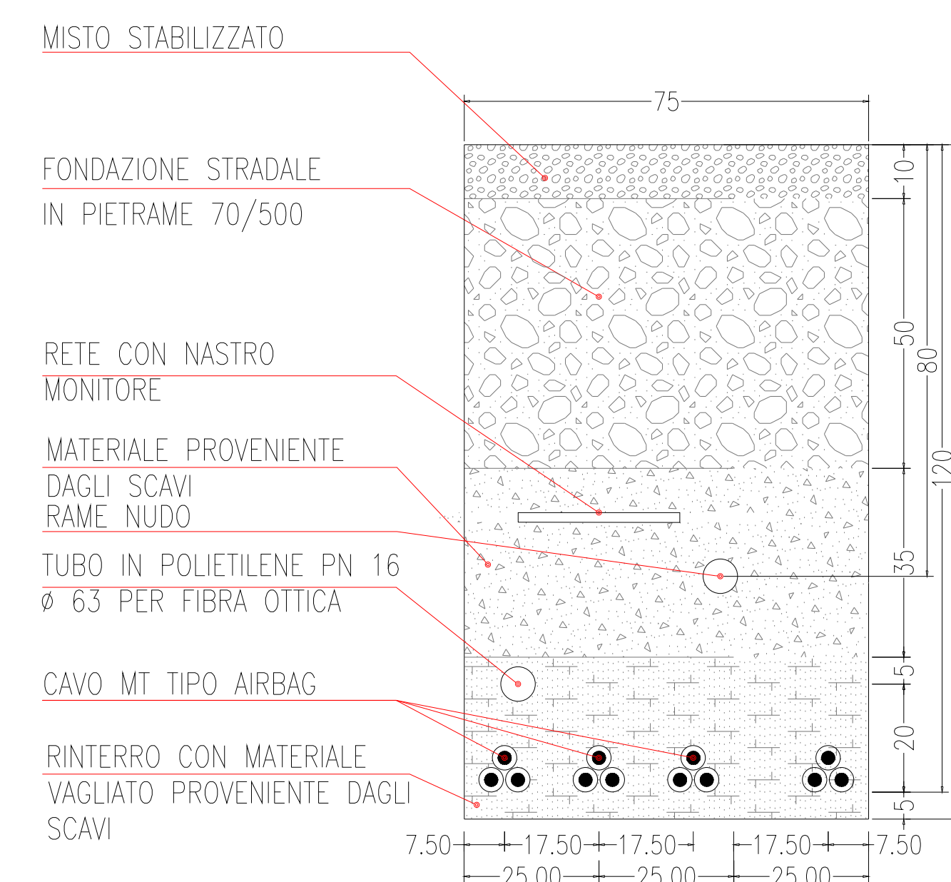
SEZIONE TIPICA C4 SU STRADA NON ASFALTATA
