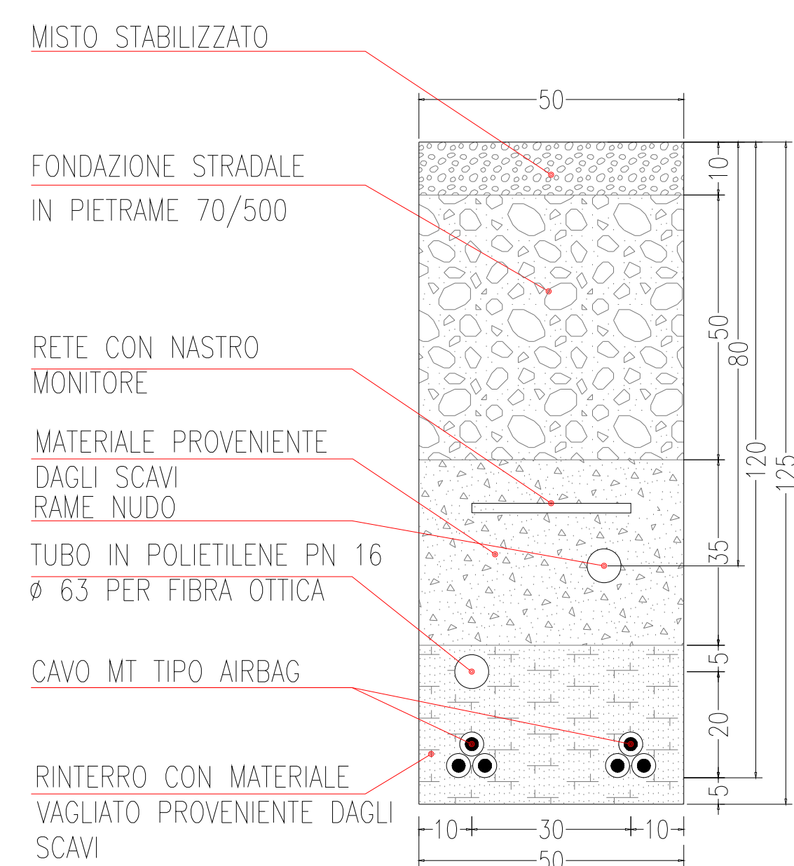
SEZIONE TIPICA C2 SU STRADA NON ASFALTATA
