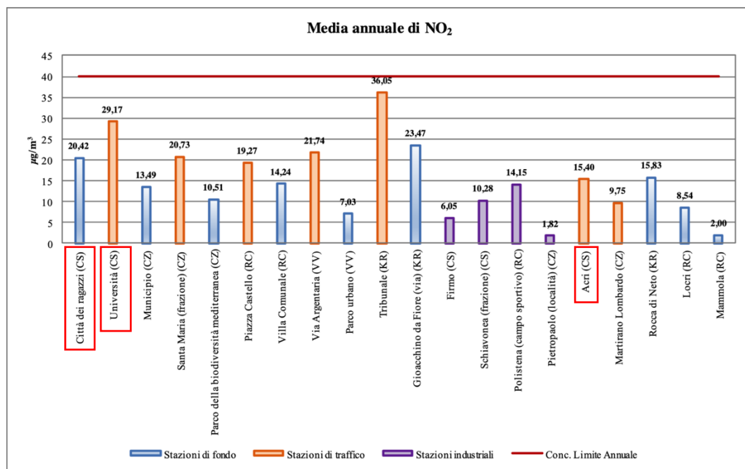
Figura 128 - Regione Calabria - NO 2 - Valori medi annuali
