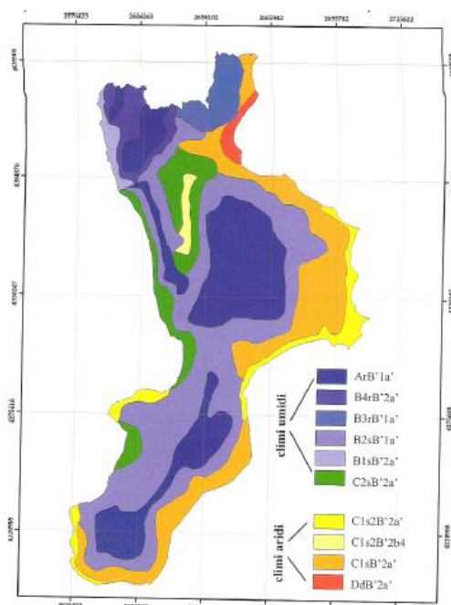
Figura 113 – Suddivisione meteoclimatica C.W. Thornthwaite per St = 150\text{mm}
