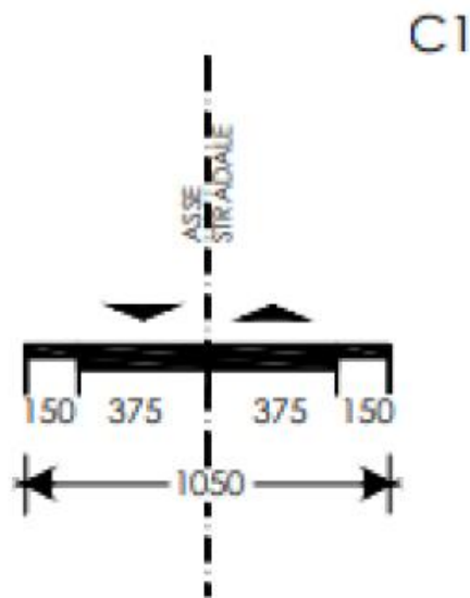
Figura 66 - Piazzafornia Tipo C1
