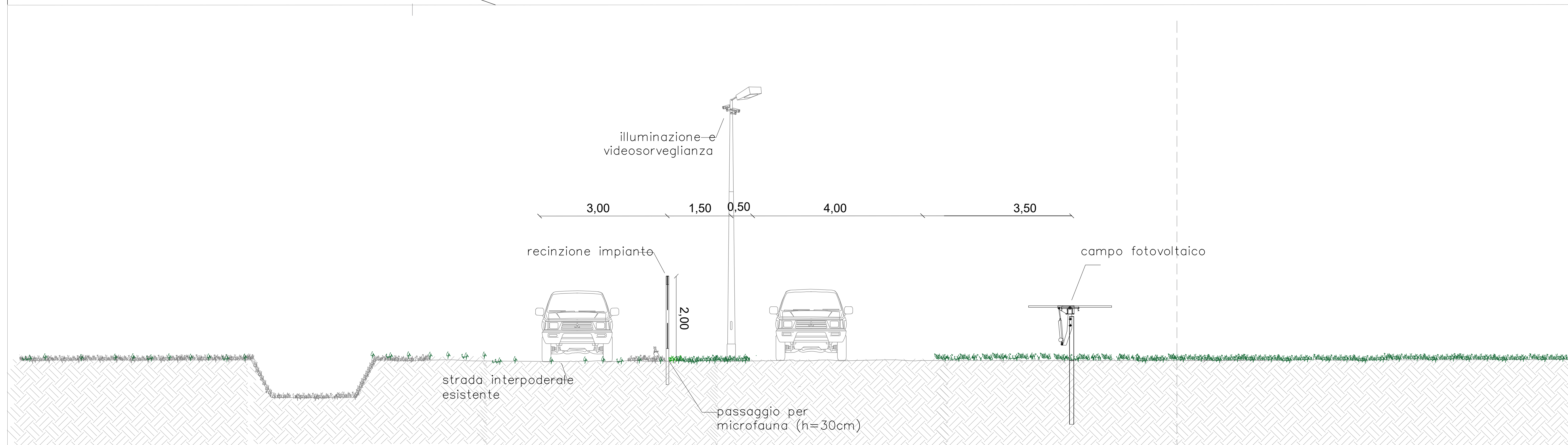
Sezione B-B' - Scala 1:100
