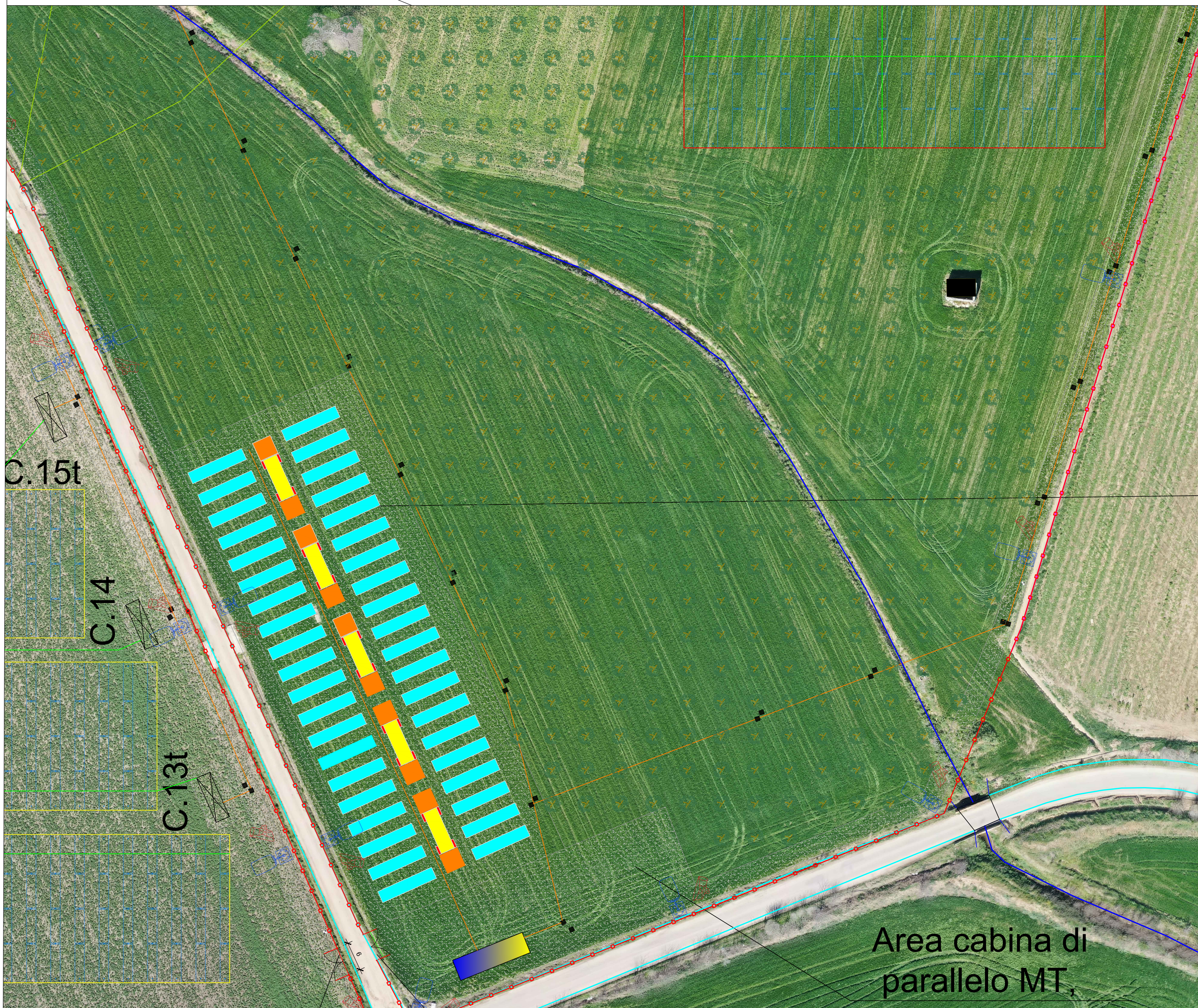
PARTICOLARE SESTO D'IMPIANTO
