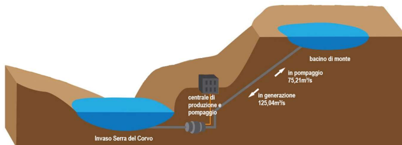
Schema funzionale impianto a pompaggio e accumulo
