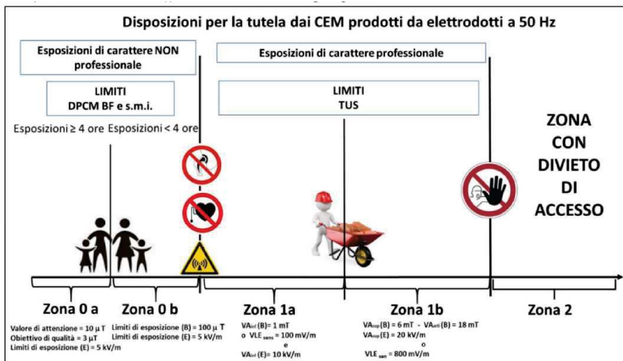
Figura 7: misure di prevenzione e protezione per la tutela dai CEM prodotti da elettrodotti a 50 Hz
