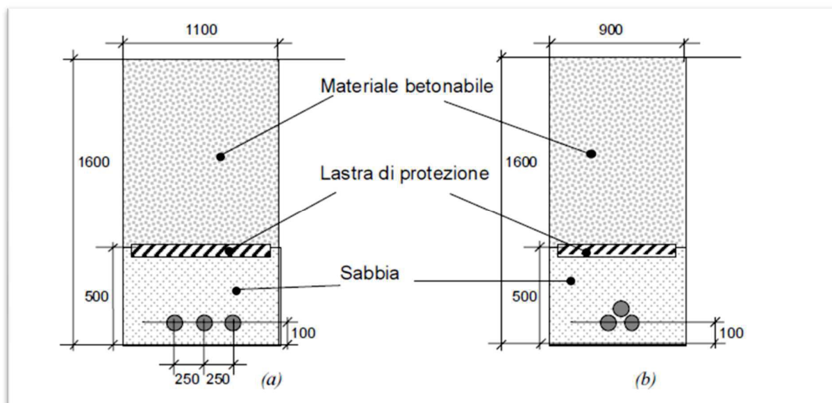
Figura 14: schermatura cavi elettrici interrati
