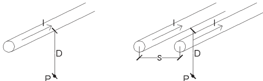
Fig. 3 - Linea Unifilare e Bifilare
