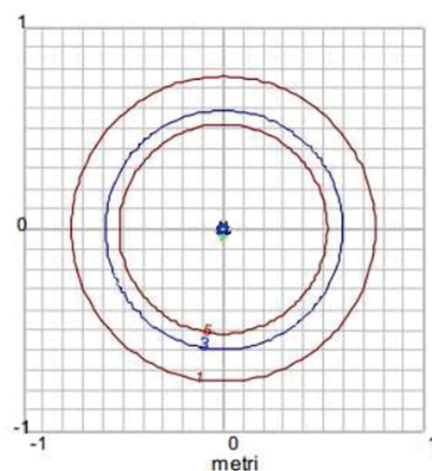
Figura 9: Curve equilivello dell’induzione magnetica generata da cavi cordati ad elica – calcoli effettuati con un modello tridimensionale che tiene conto del passo d’elica.
