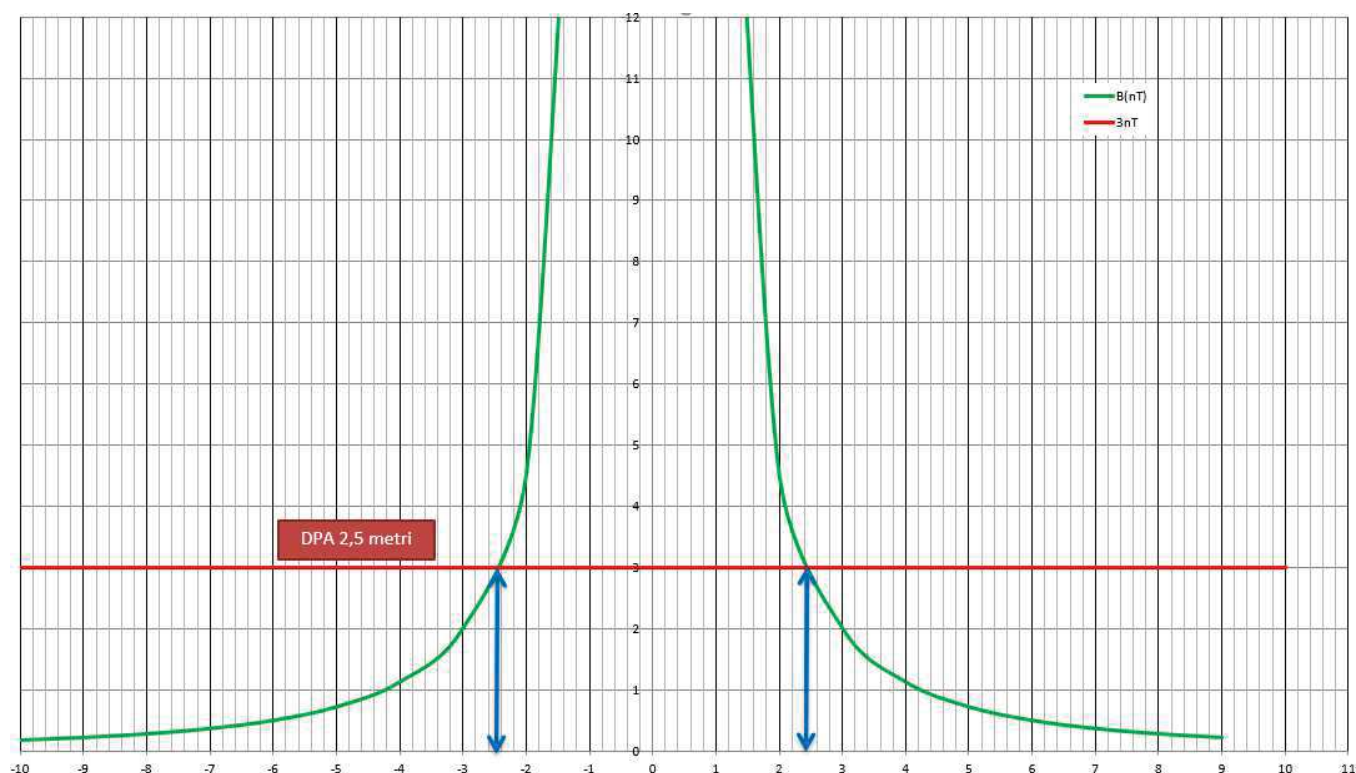
Figura 11 - Andamento del campo di induzione magnetica prodotto dal cavidotto AT in funzione della distanza dall'asse dei conduttori
