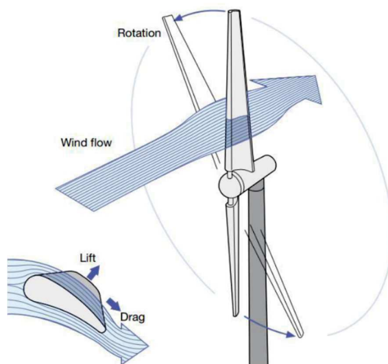
Figura 5: portanza aerodinamica sulle pale di un aerogeneratore
