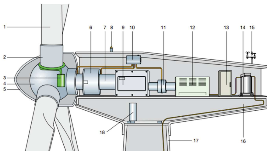
Figura 6: principali componenti di una turbina eolica
