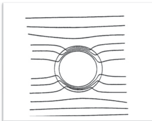
Figura 13: andamento qualitativo della deformazione delle linee di forza di un campo magnetico uniforme per effetto di un nucleo in materiale ferromagnetico
