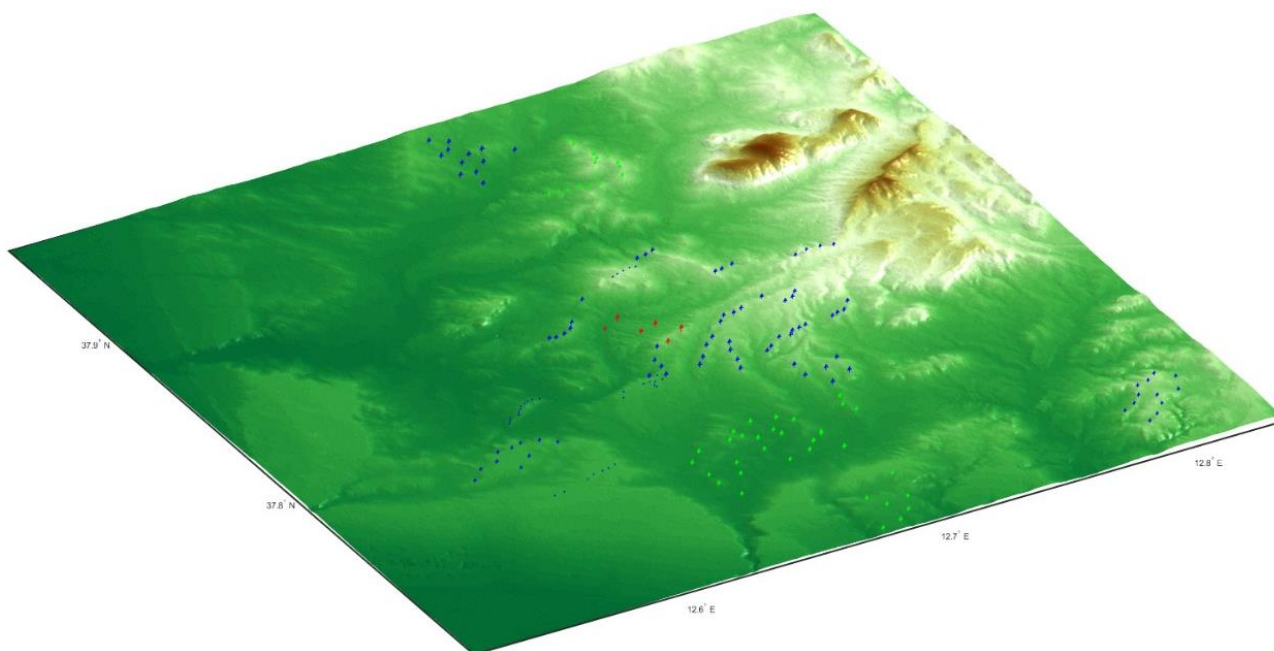
Figura 1-12 Modello digitale del terreno 3D sviluppato su un raggio di 14 km e rappresentazione parchi eolici esistenti/autorizzati (blu) in fase di autorizzazione (verde), progetto (rosso)
