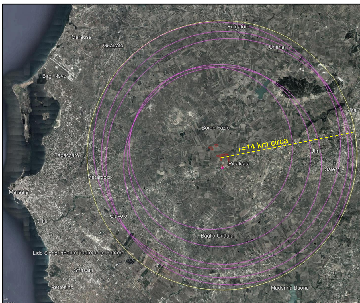
Figura 1-1. Nuova area vasta di studio ai fini degli impatti cumulativi (cerchio giallo r=14 km). In rosso i lotti catastali di intervento; in magenta i cerchi con r=50 H_{max} di ciascun aerogeneratore in progetto.
