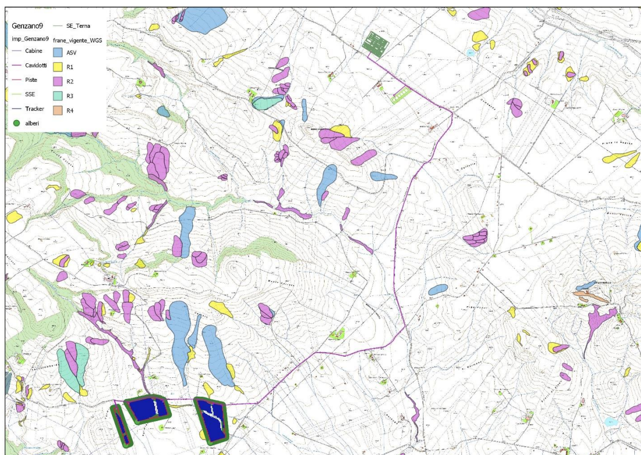
Figura 3.2. – Stralcio Carta delle Frane: localizzazione impianto e sottostazioni.
