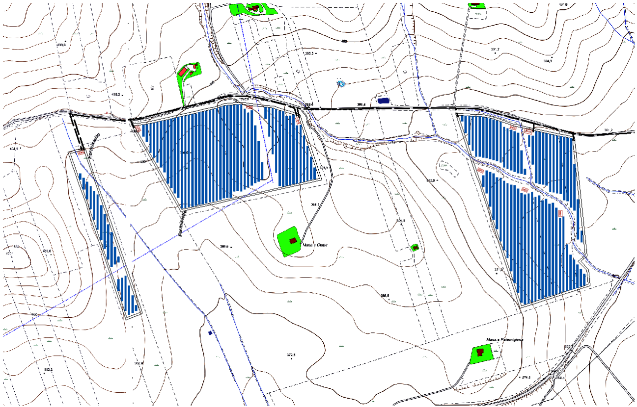
Figure 4.5 Progetto dell'impianto FV su CTR – dettaglio (base scala 1:5.000)
