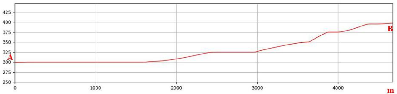
Sezione morfologica del terreno- Punto di presa n°7
