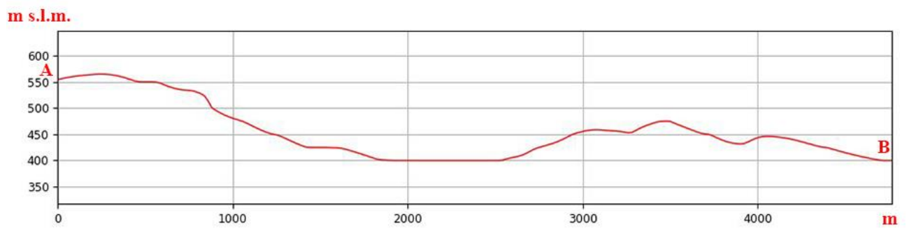
Sezione morfologica del terreno- Punto di presa n°4
