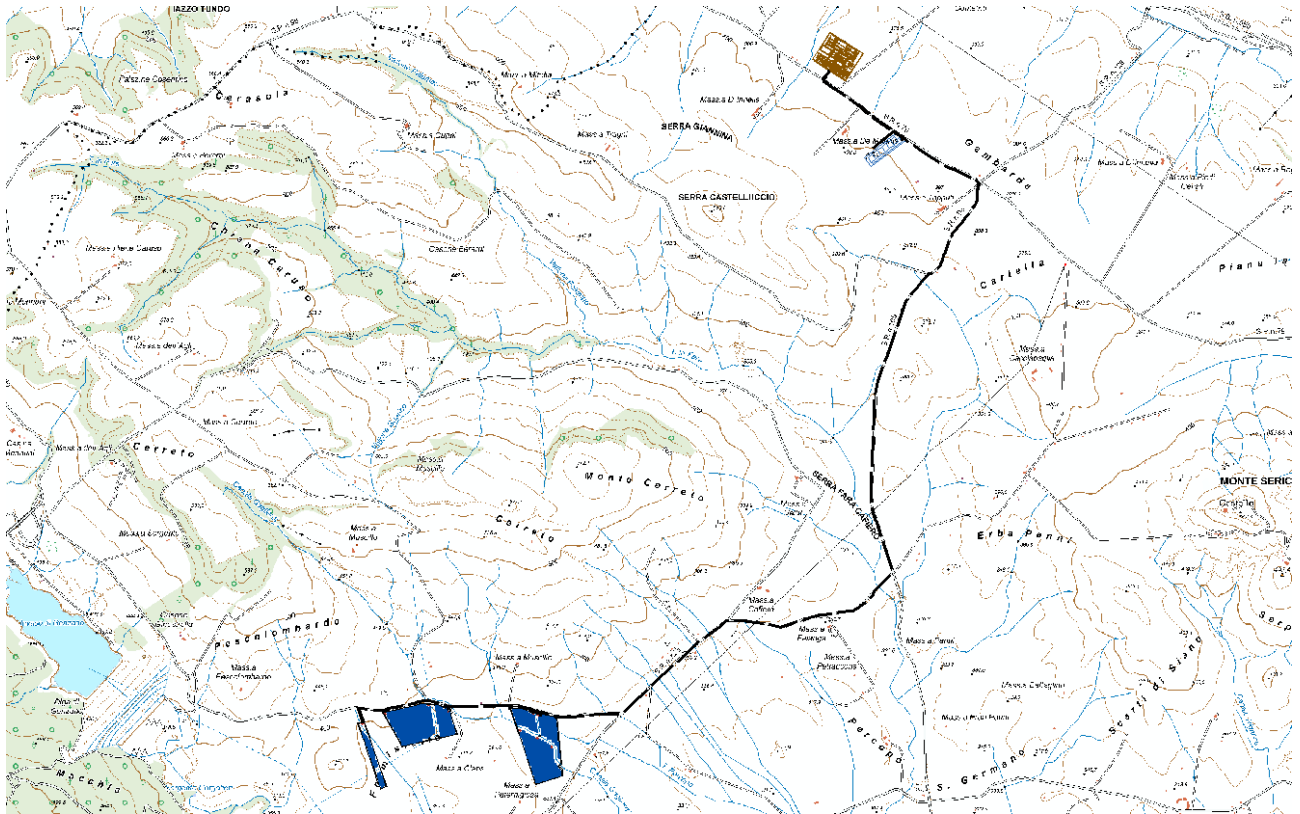
Figure 4.3 Progetto dell'impianto FV su CTR (base scala 1:25.000)
