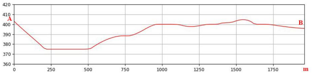
Sezione morfologica del terreno- Punto di presa n°9
