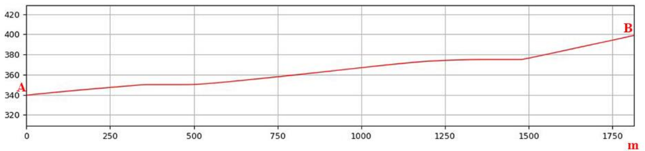
Sezione morfologica del terreno- Punto di presa n°8
