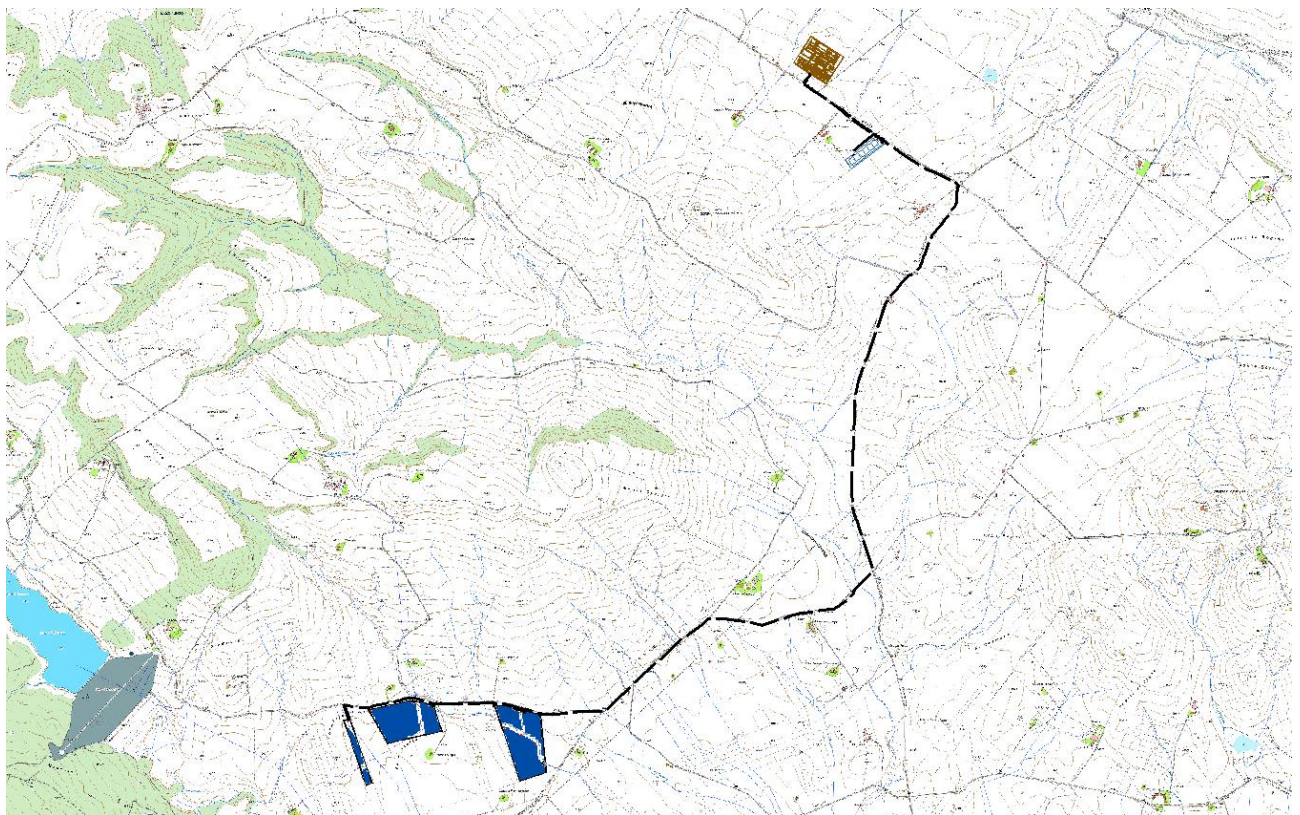
Figure 4.4 Progetto dell'impianto FV su CTR (base scala 1:10.000)
