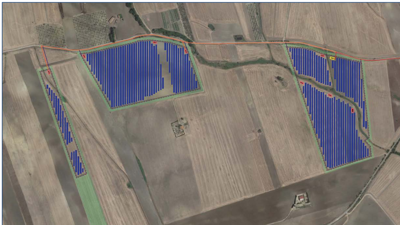
Figura 2 - Inquadramento Ortofoto-Catastale dell'area di studio con Area Impianto FV
