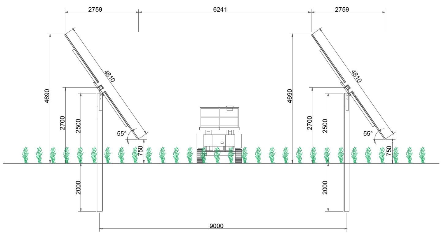
Figura 13 - Struttura di supporto con distanza tra i tracker.
