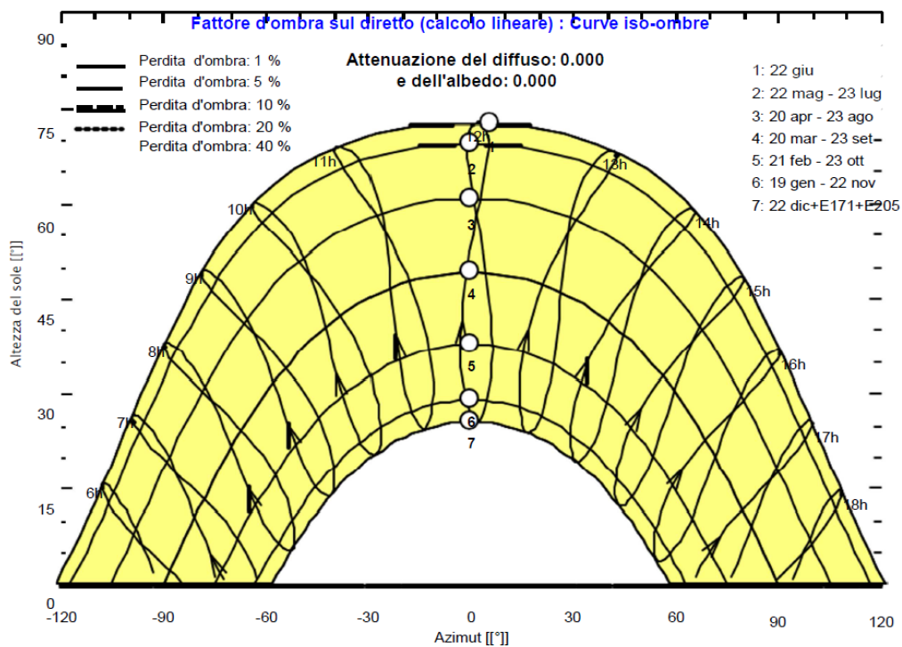
DIAGRAMMA ISO-OMBRE
