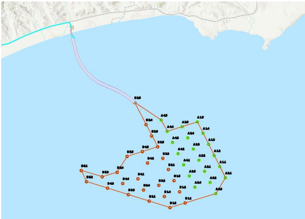
Figura 1:1: Vista installazioni marine del parco Minervia Energia
