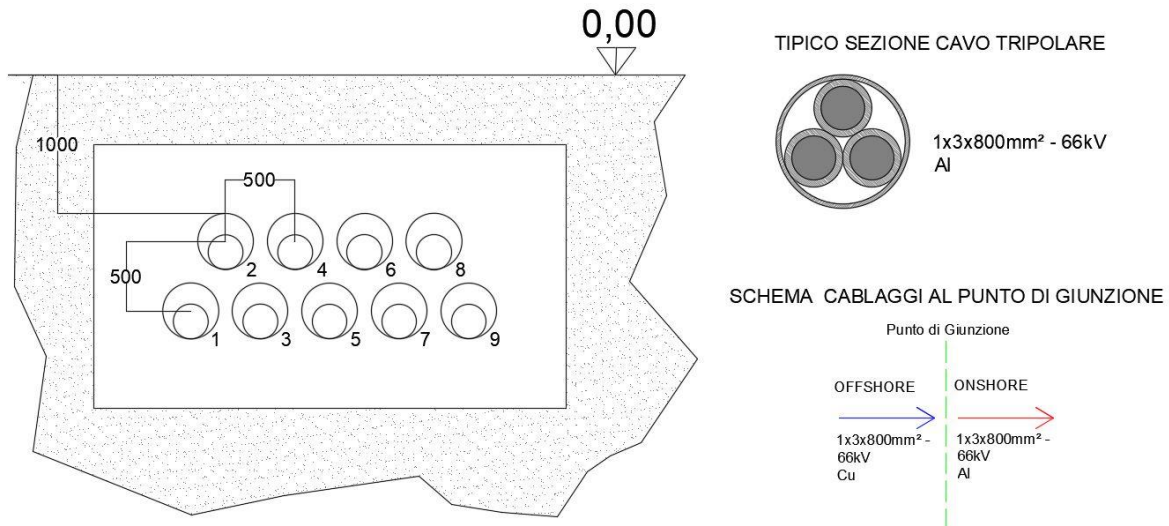
Figura 3:12: Configurazione cavi terrestri 66kV
