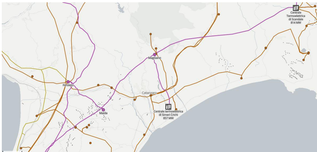
Figura 2:1: Schema delle linee in AT della Calabria (380 kV in viola e 220 kV in arancione)
