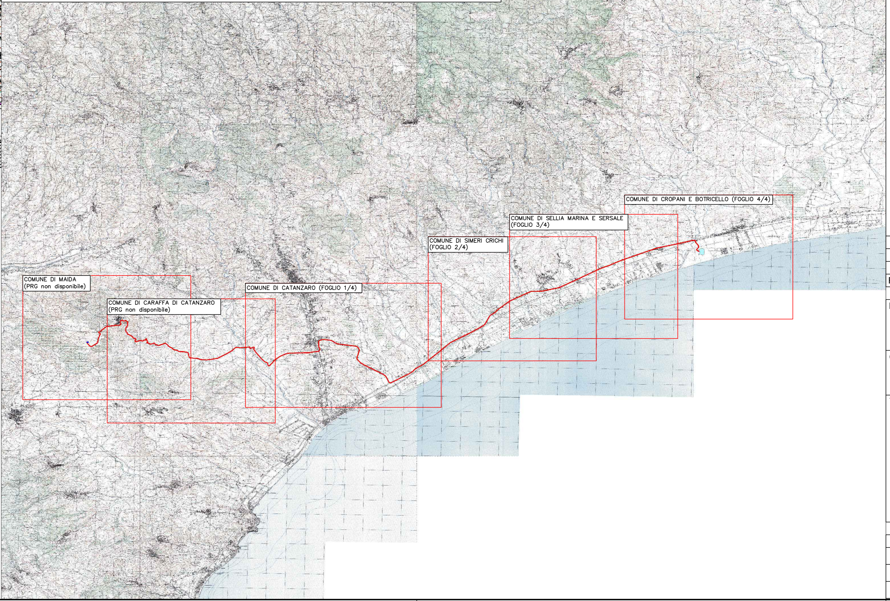
KEYPLAN – TRACCIATO CAVIDOTTO INTERRATO
