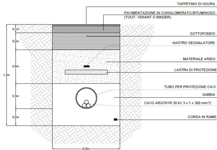
Fig 4– Sezione tipo y-y' cavidotto esterno MT verso SE
