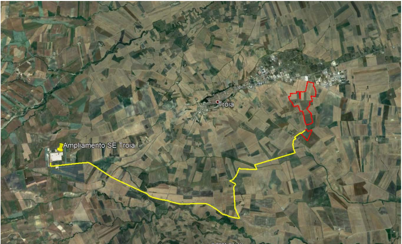
Fig. 3– Tracciato cavidotto MT verso SE
