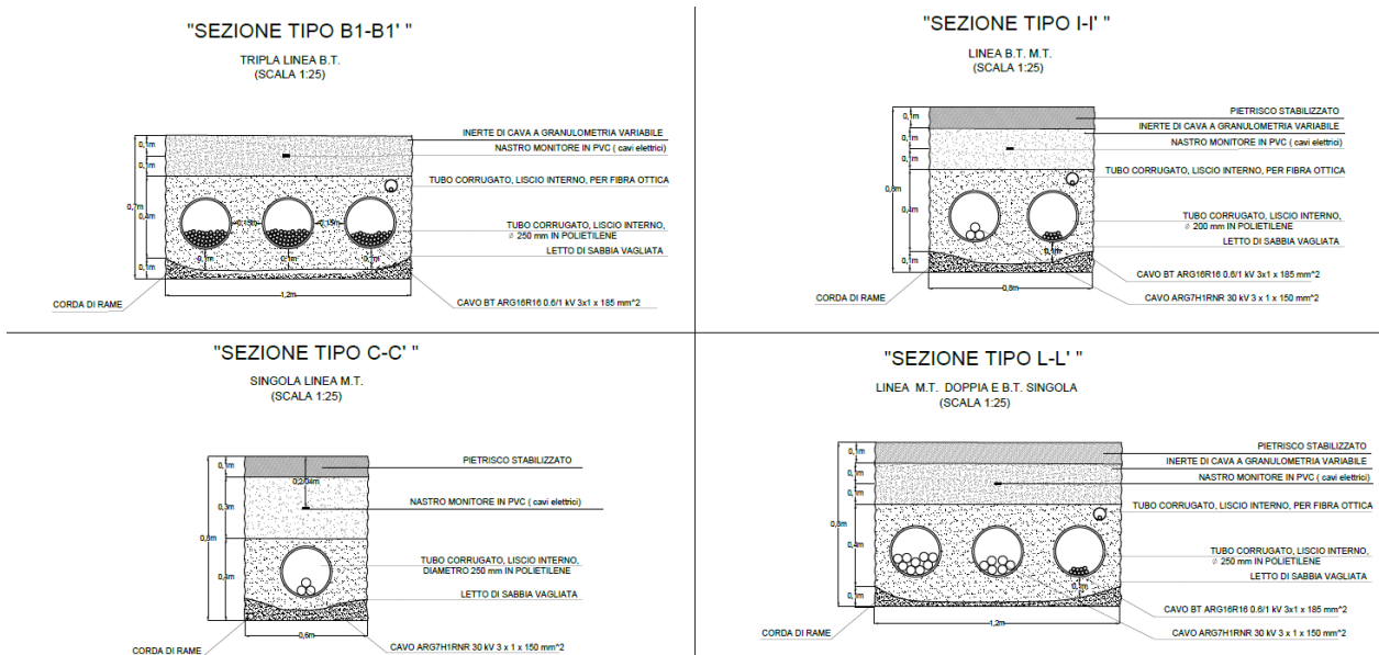
Fig. 2– Sezioni tipo cavidotti interni BT ed MT
