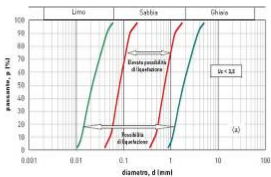
Figura 13 A Fusi granulometrici suscettibili a liquefazione con U < 3.5
