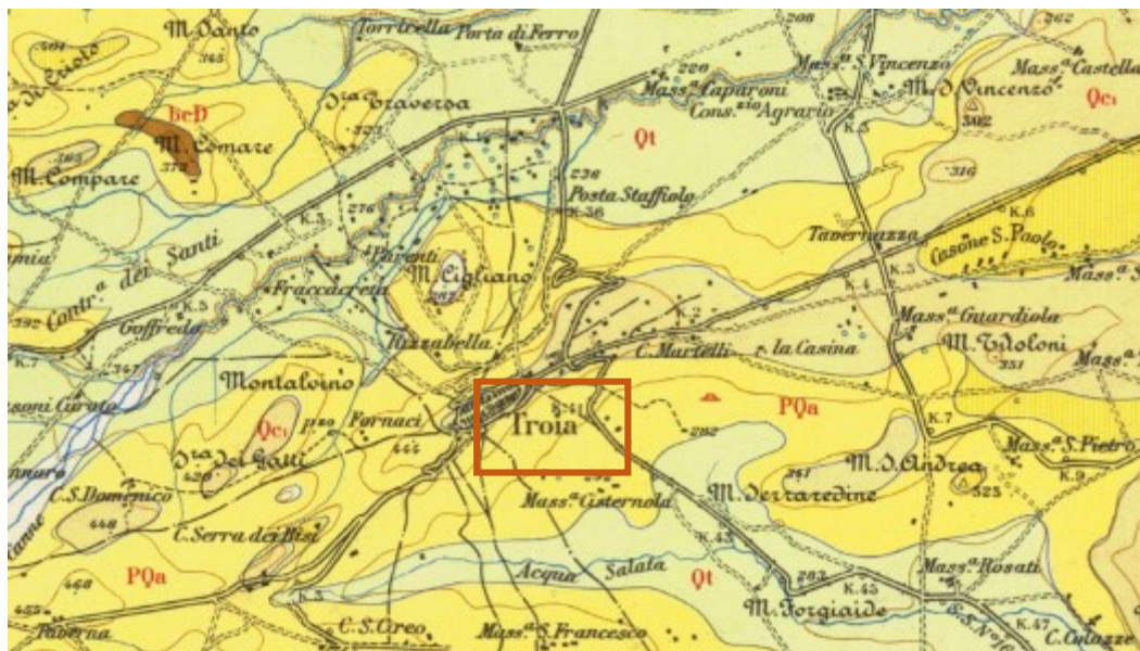
Figura 4- Stralcio del Foglio 163 Lucera della Carta Geologica d'Italia alla scala 1:100.000
