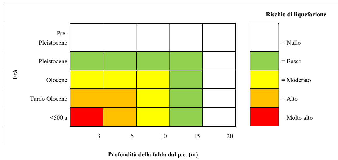
Figura 11- Rischio liquefazione in funzione dell'età del deposito e della profondità della falda, tratta da "La liquefazione dei terreni" Giulio Riga, 2007, ridisegnata – Dario Flaccovio Editore.
