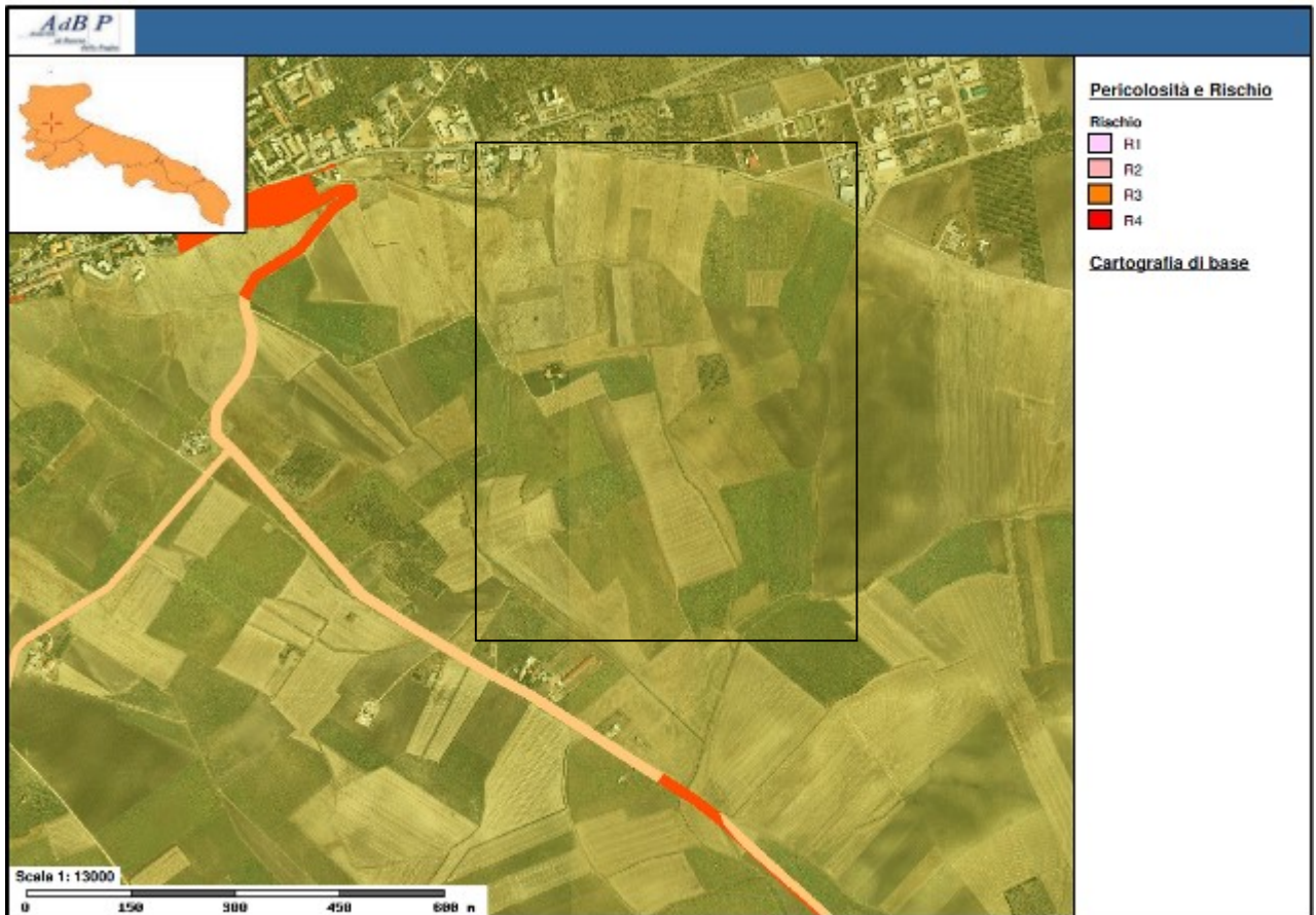
Figura 16 - PAI stralcio carta del Rischio con legenda. http://webgis.adb.puglia.it/gis/map_default.phtml
