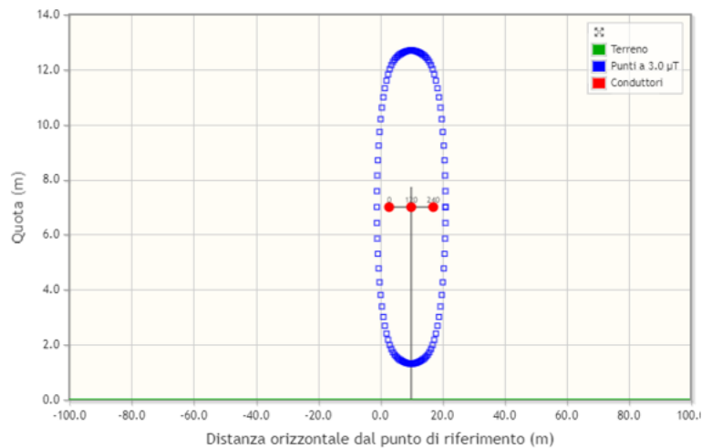
Figura 63- Stima distanza orizzontale
