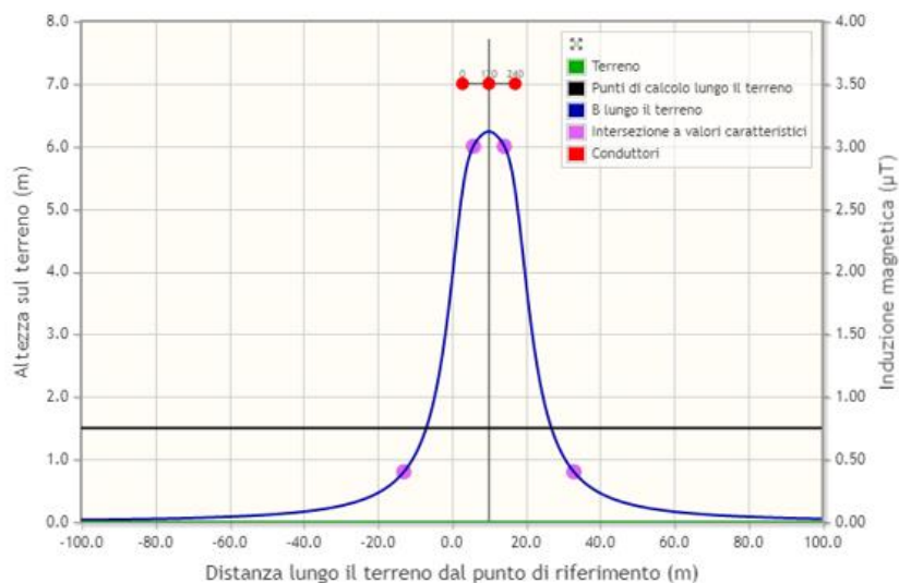
Figura 62 - Stima Campo elettromagnetico Stazione AT
