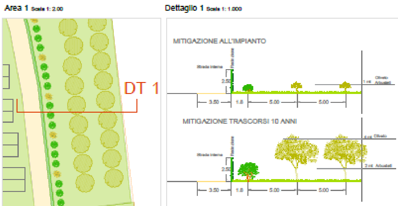
Figura 68 - Esempio, particolare mitigazione piastra 1
