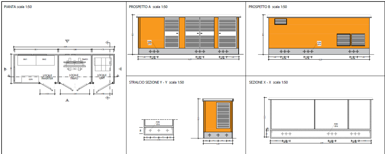
Figura 15 - Cabina di campo
