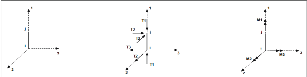
Figura 11 - Sistema di riferimento locale per i pilastri
