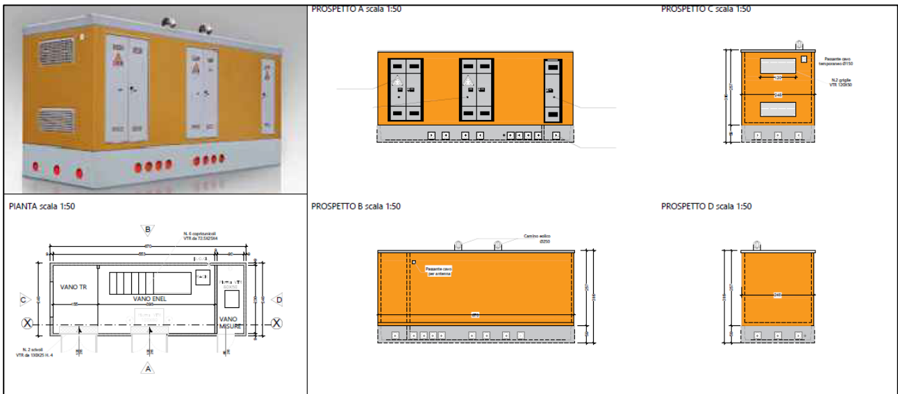
Figura 14 - Cabina Enel
