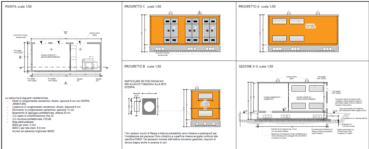
Figura 13 - Cabina di sezionamento utente
