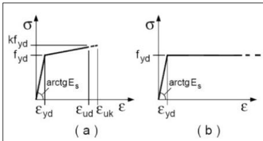
Figura 6 - Diagrammi costitutivi acciaio
