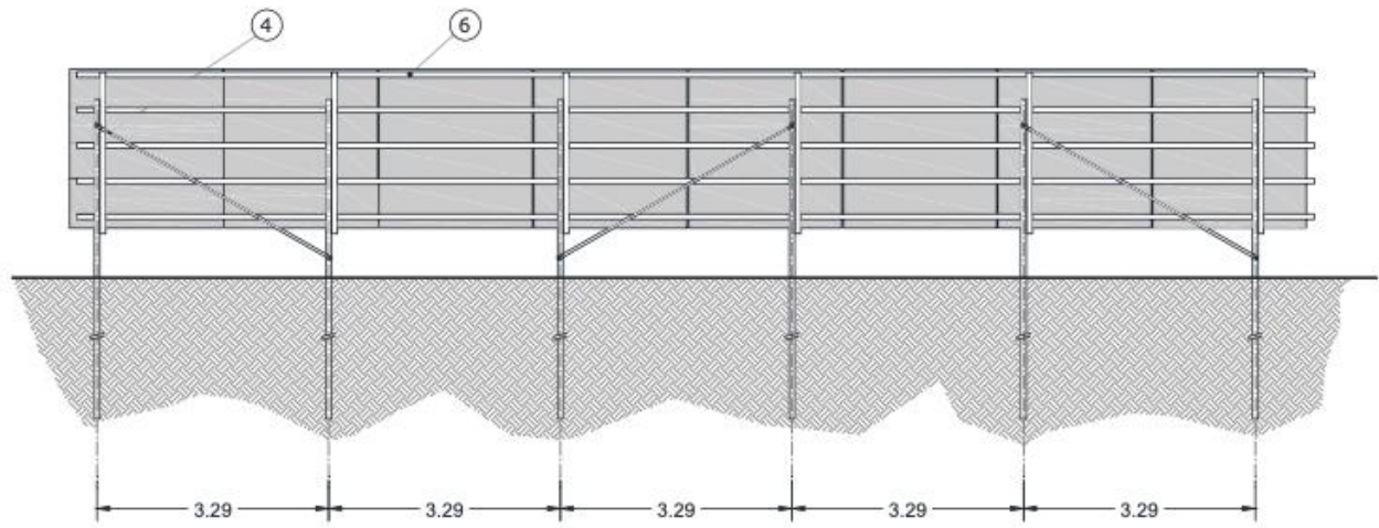
Figura 4 – Rappresentazione della struttura di supporto (posteriore)
