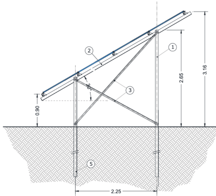
Figura 3 – Rappresentazione della struttura di supporto (laterale)
