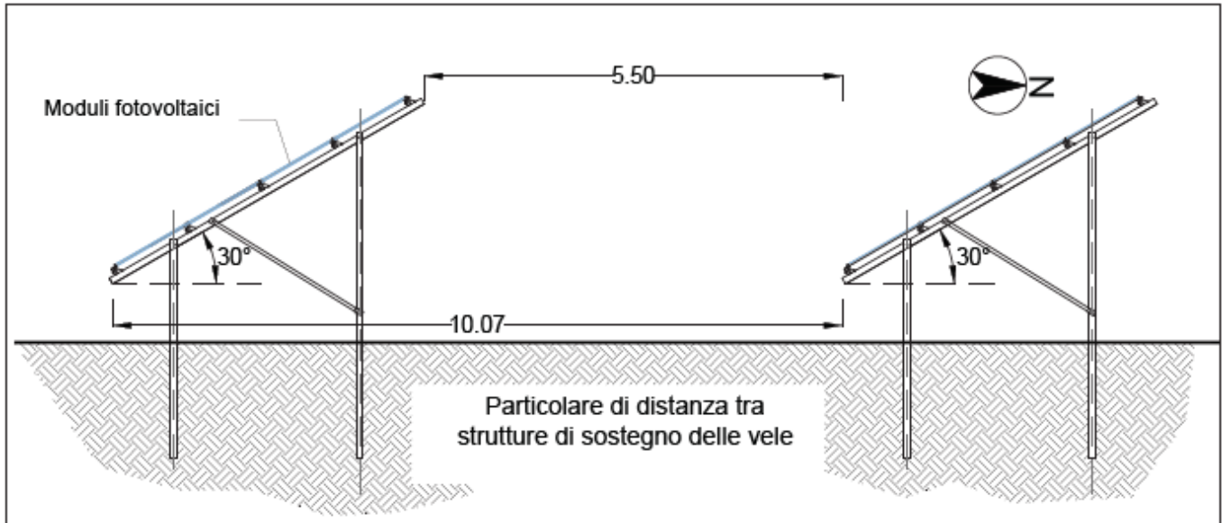
Fig.2- Particolare di struttura serra con moduli fotovoltaici prevista
