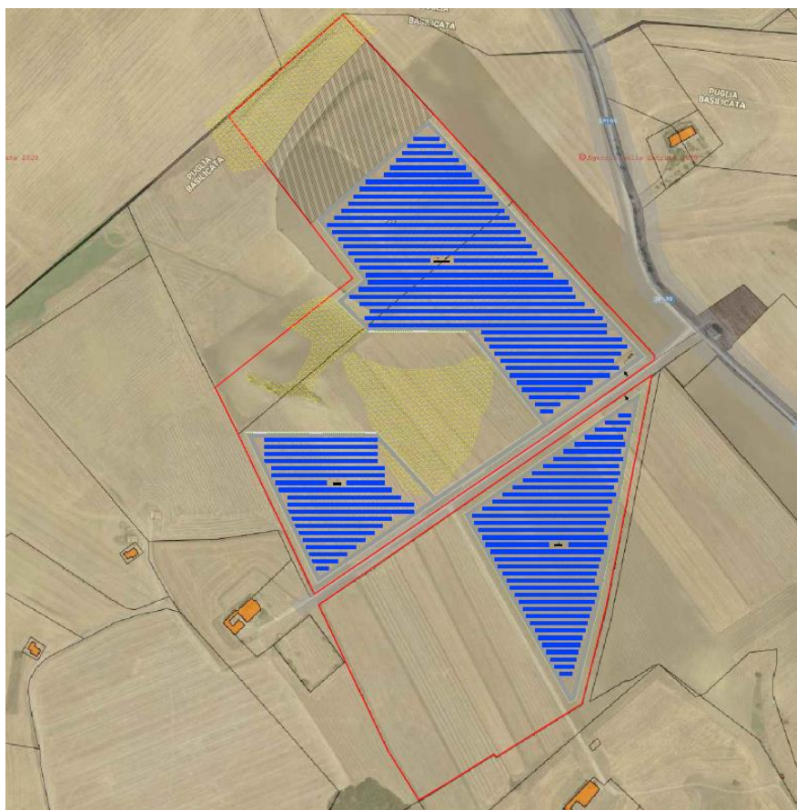
Fig.1- Impianto con indicazione dei 10 lotti e relative serre con fotovoltaico
