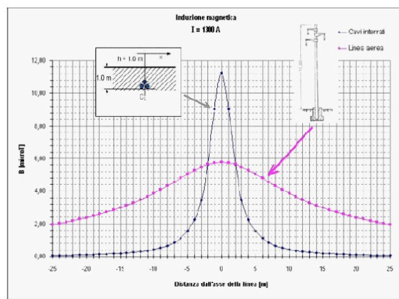
Figura 1: Attenuazione dell'induzione magnetica dovuta all'interramento dei cavi
