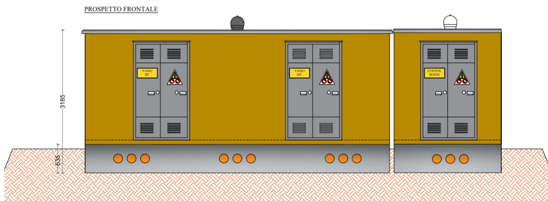
Figura 37 – Cabina
