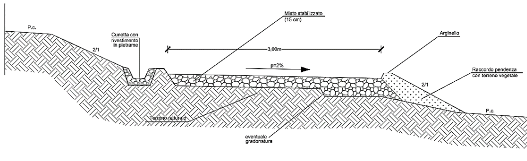
Figura 41 - Sezione tipo strade interne al sito, tipologia a mezza costa (Fonte: ns elaborazione)
