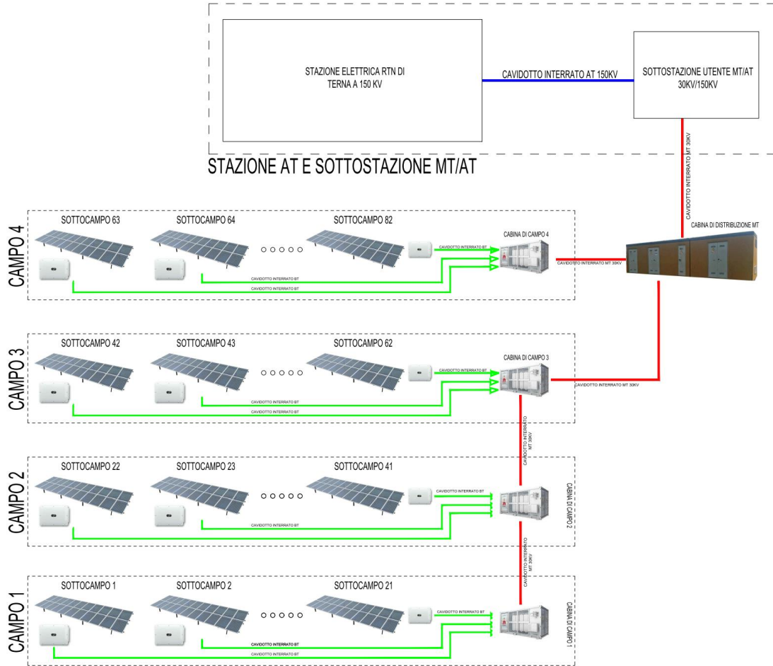
Figura 43 – Schema delle connessioni elettriche
