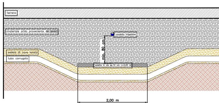
Figura 45 – Interferenze cavidotto
