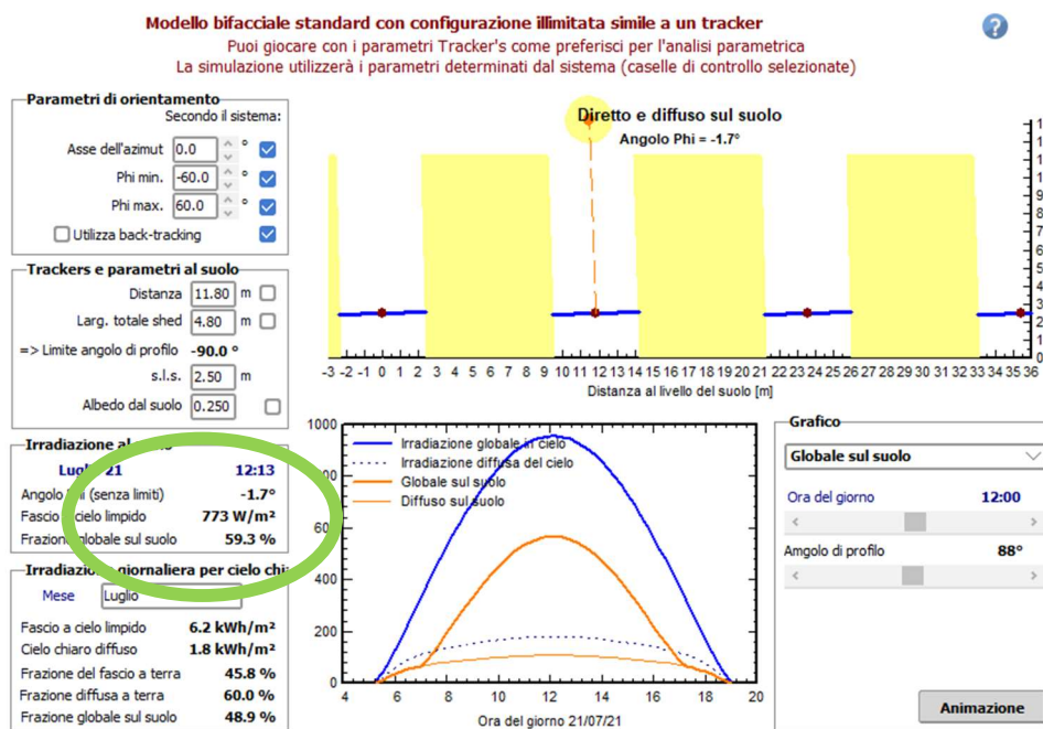
73 – esempio del calcolo dell'irradiamento relativo al mese di luglio
