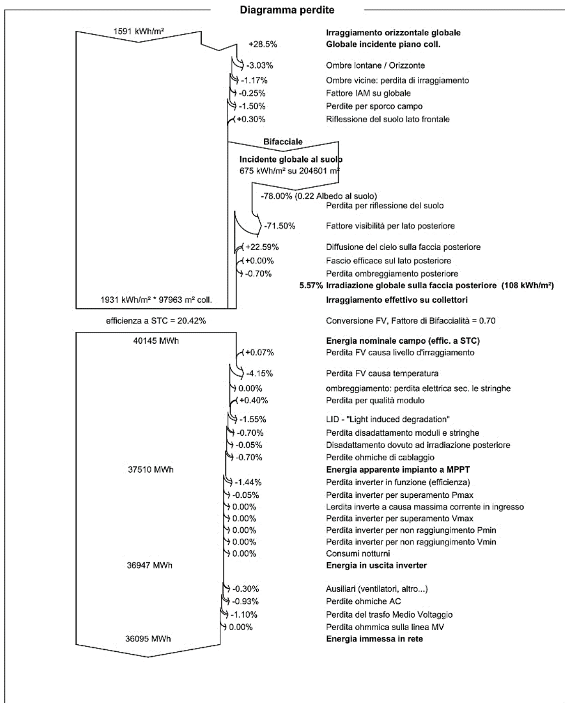
Figura 2- Calcoli PVsyst
