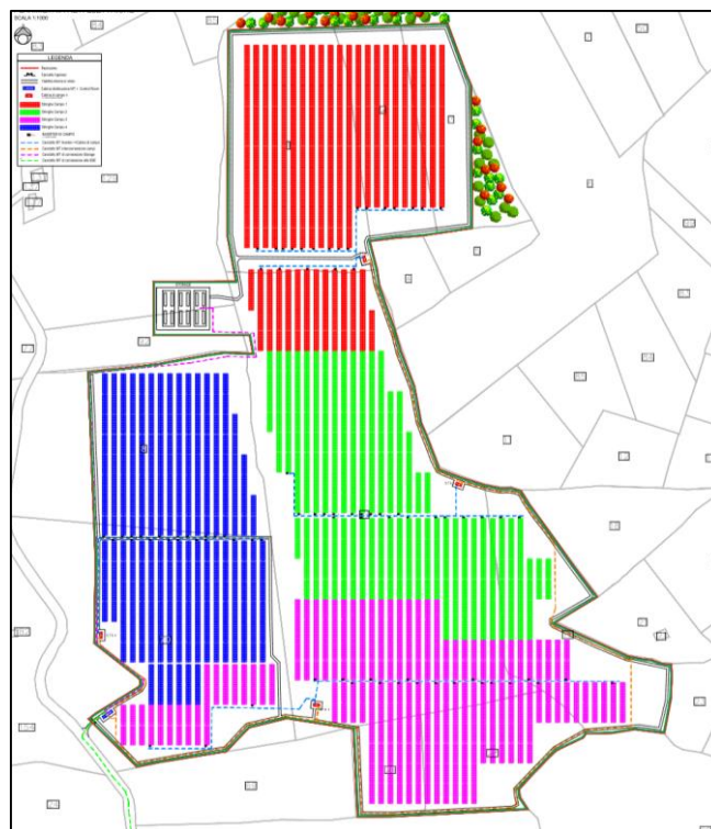
Figura 1 - Planimetria impianto agrivoltaico
