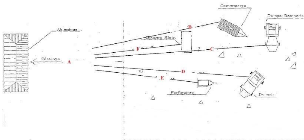
Figura 4 - distanziamento medio macchinari dal recettore sensibile più vicino
