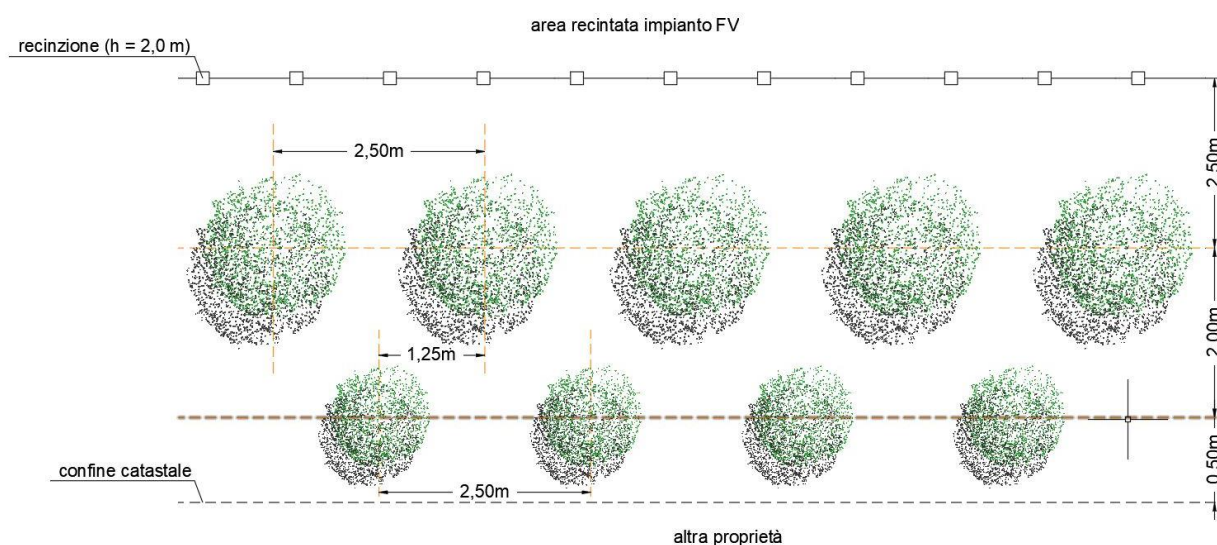
Figura 4.2. – Siepe polispecifica (planimetria di progetto).
