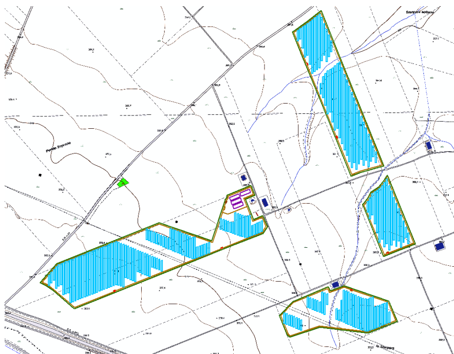
Figura 2.4b. – Area di progetto con indicazione del posizionamento dei moduli fotovoltaici.
