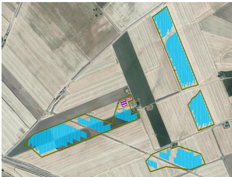
Figura 2.4a. – Area di progetto con indicazione del posizionamento dei moduli fotovoltaici.
