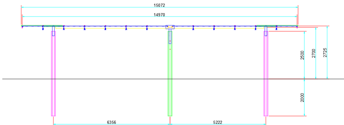
Figura 2.3 – Sezione longitudinale.
