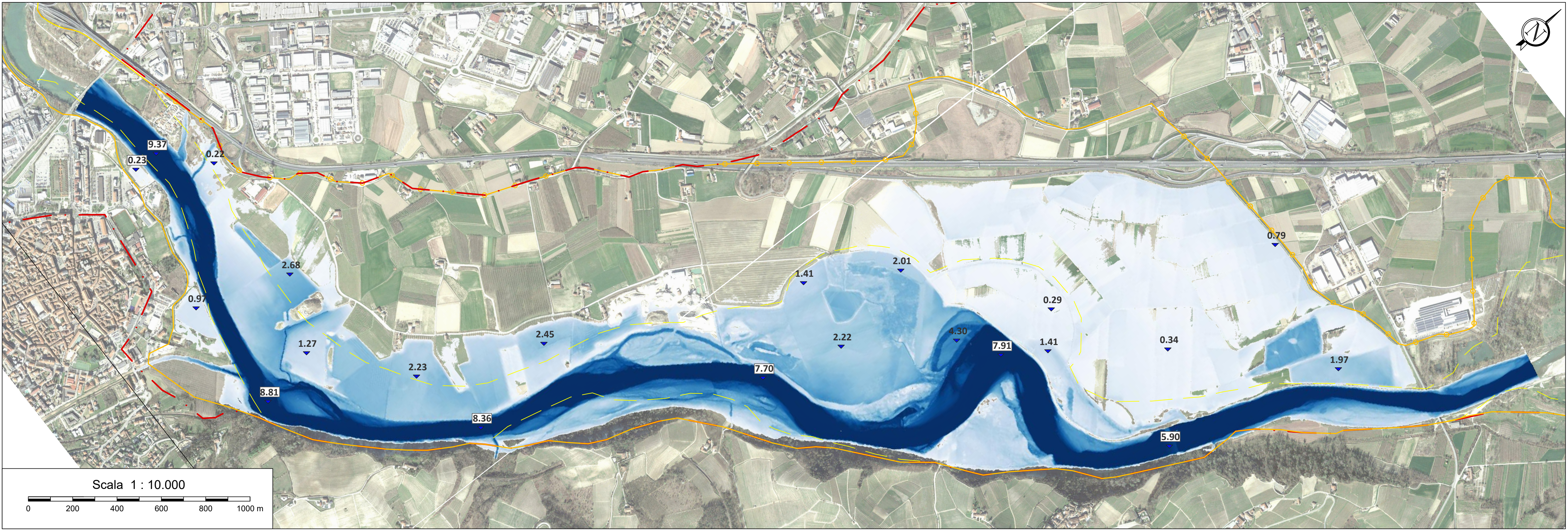
CARTA DELLE AREE DI ESONDAZIONE ALLO STATO DI PROGETTO PER LA PIENA TR 200 ANNI Base carta: ORTOFOTO SATELLITARE 2021
