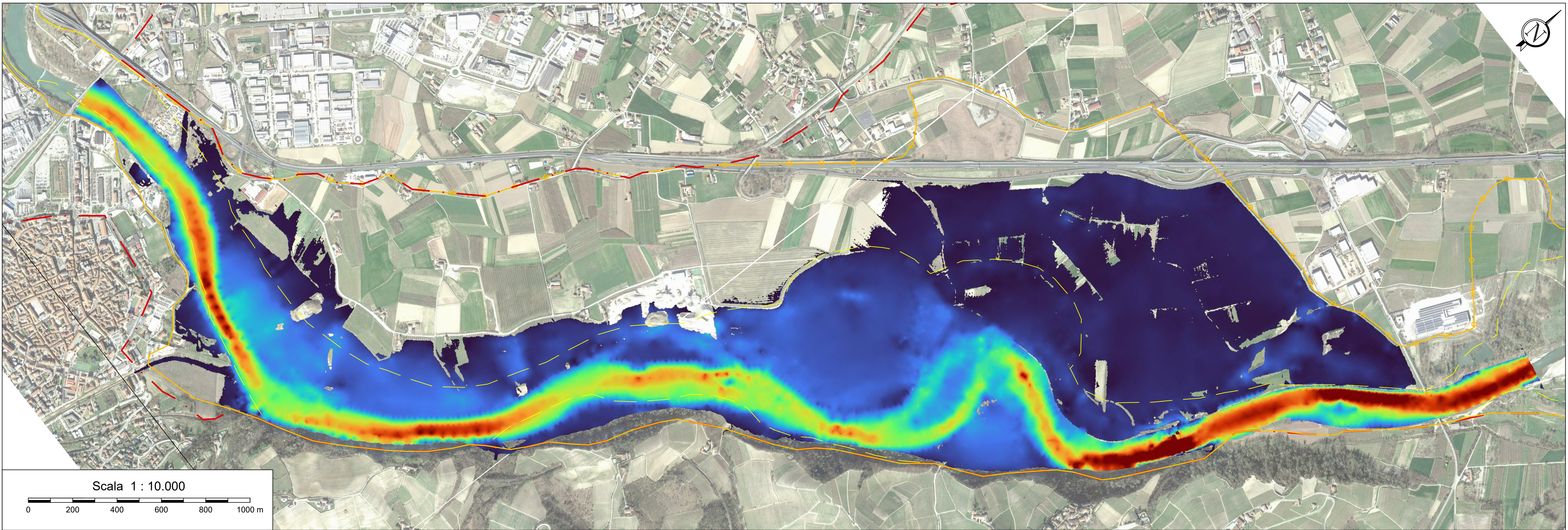
CARTA DELLA DISTRIBUZIONE DELLE VELOCITA' DI DEFLUSSO ALLO STATO DI PROGETTO PER LA PIENA TR 200 ANNI Base carta: ORTOFOTO SATELLITARE 2021
