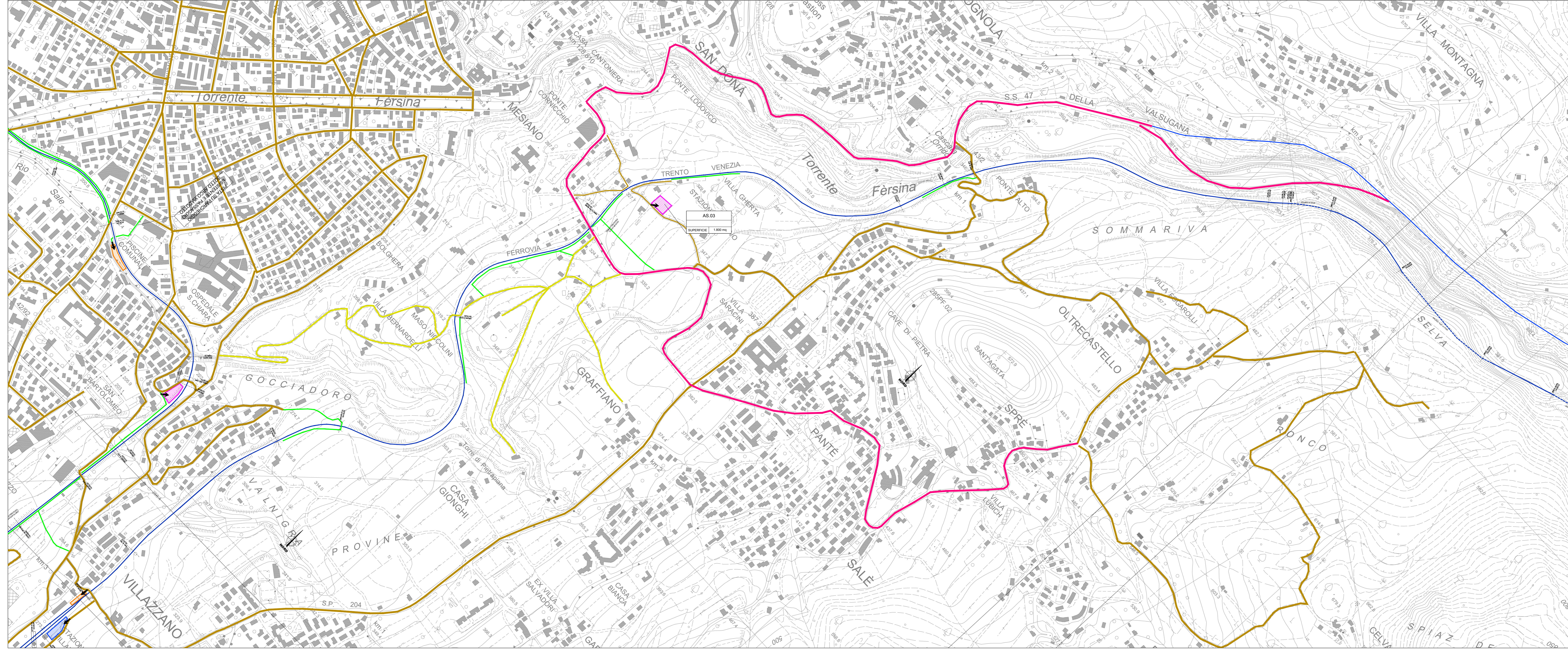
PLANIMETRIA DI CANTIERIZZAZIONE RIQUADRO 1.3 - Scala 1:5000
