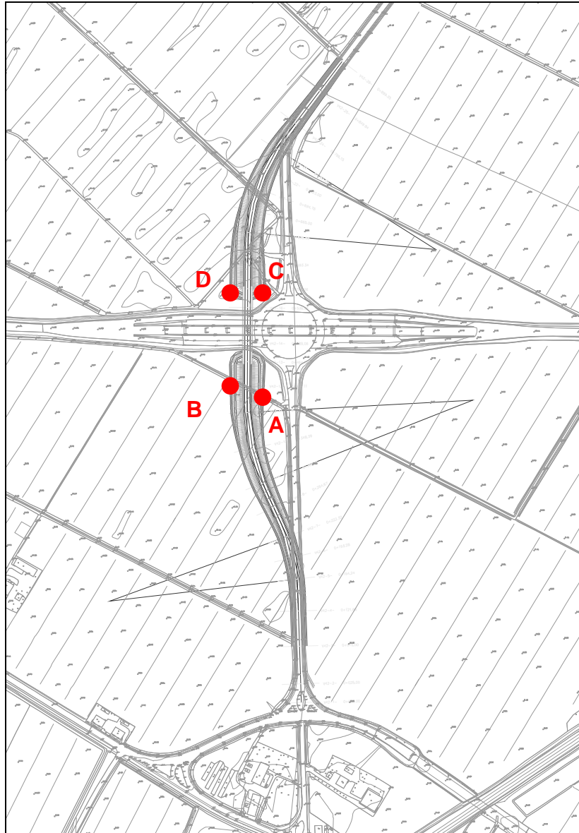
Figura 8.1 – Indicazioni dei punti di scarico più significativi sottoposti a verifica
