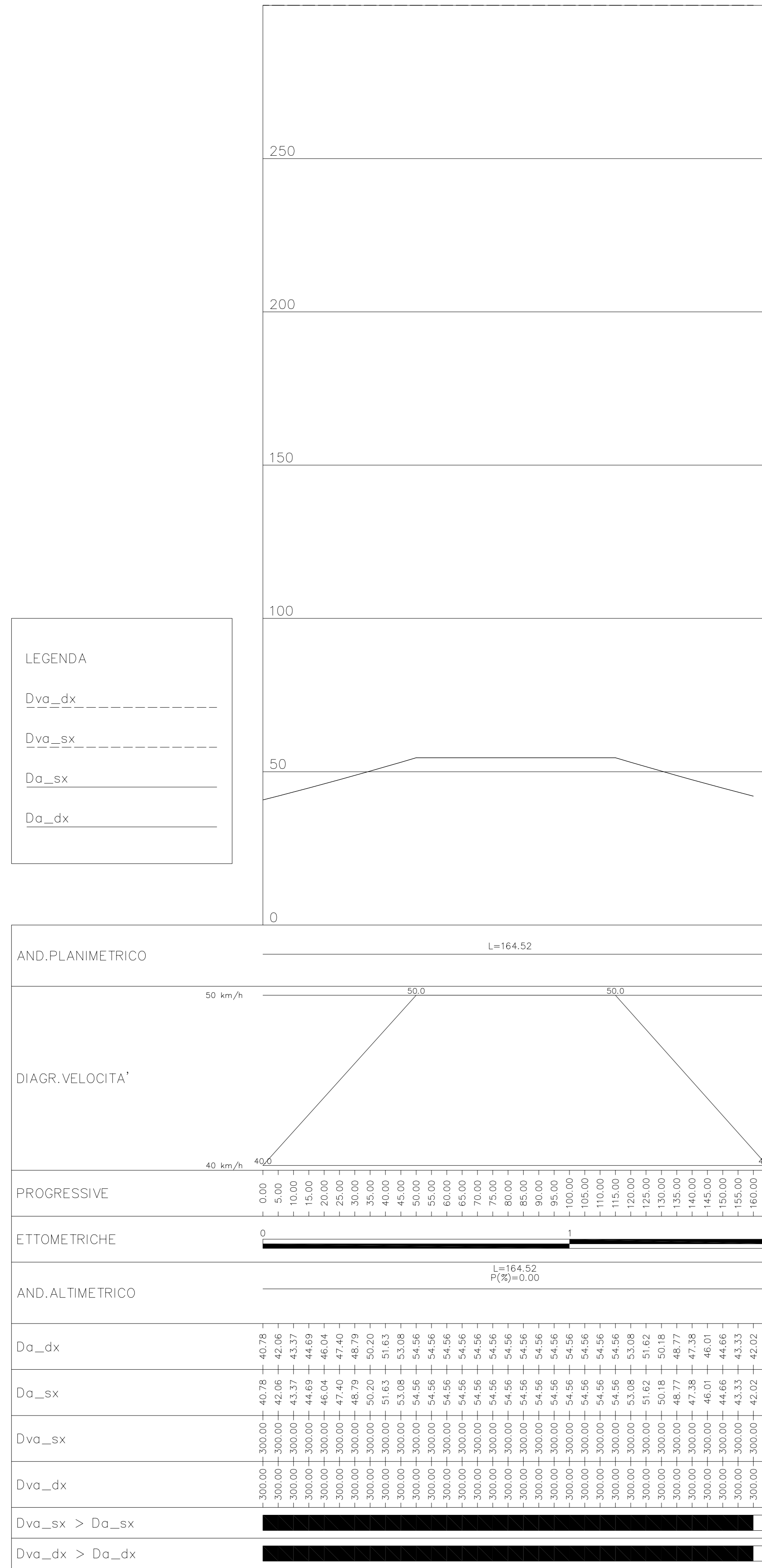
DIAGRAMMA DI VISUALE LIBERA E DI VELOCITA' X= 1:1000/ Y= 1:1000 STP VIA IMPERIALE CAMURANA
