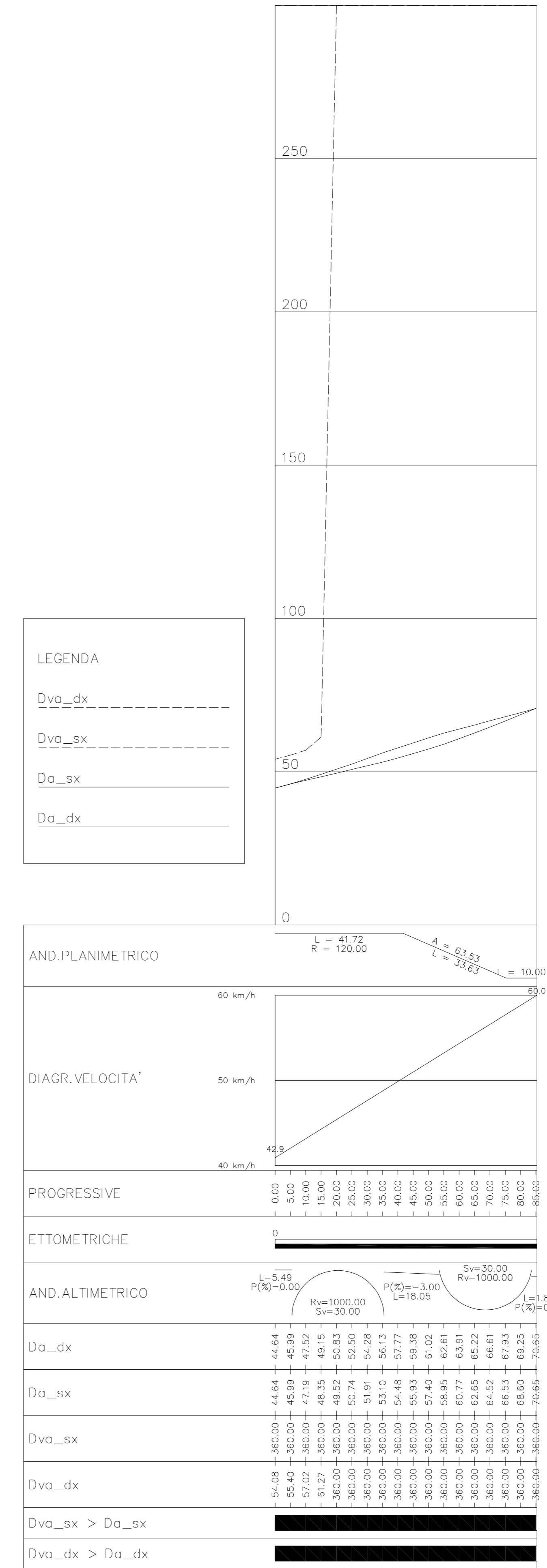
DIAGRAMMA DI VISUALE LIBERA E DI VELOCITA' X= 1:1000/ Y= 1:1000 RAMO A
