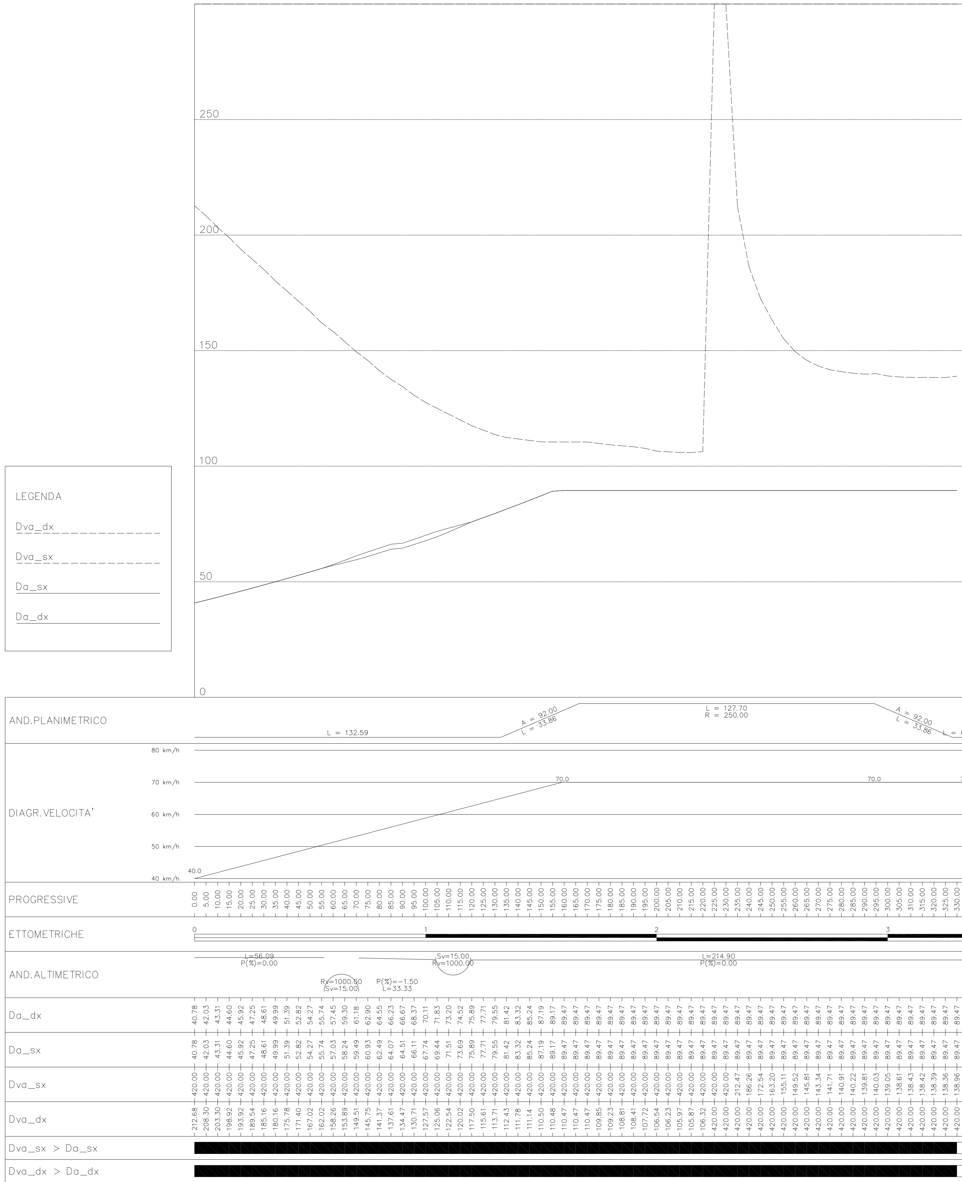
DIAGRAMMA DI VISUALE LIBERA E DI VELOCITA' X= 1:1000/ Y= 1:1000 RAMO B
