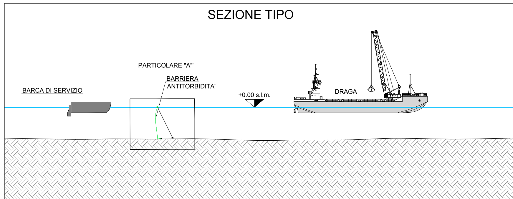
Dispiegamento della barriera antitorbidità
