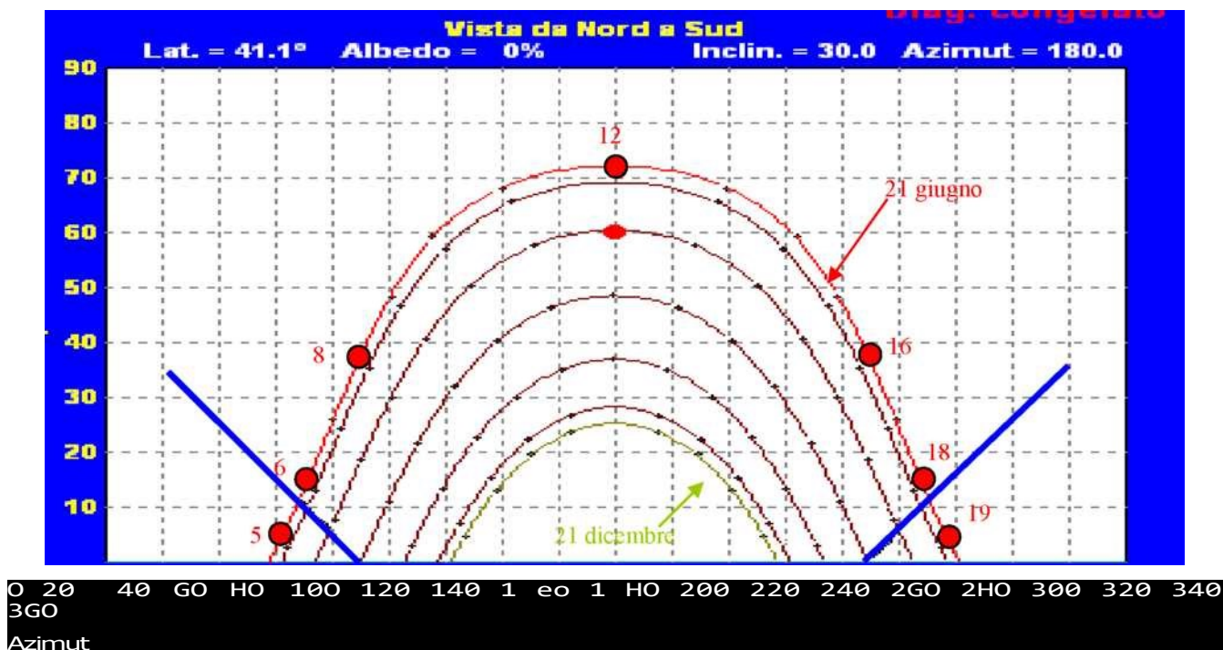
Figura 1 - Diagrammi solari della città di Bari e orari di illuminazione dei moduli FV (Elaborazione con Software Sunsim)
