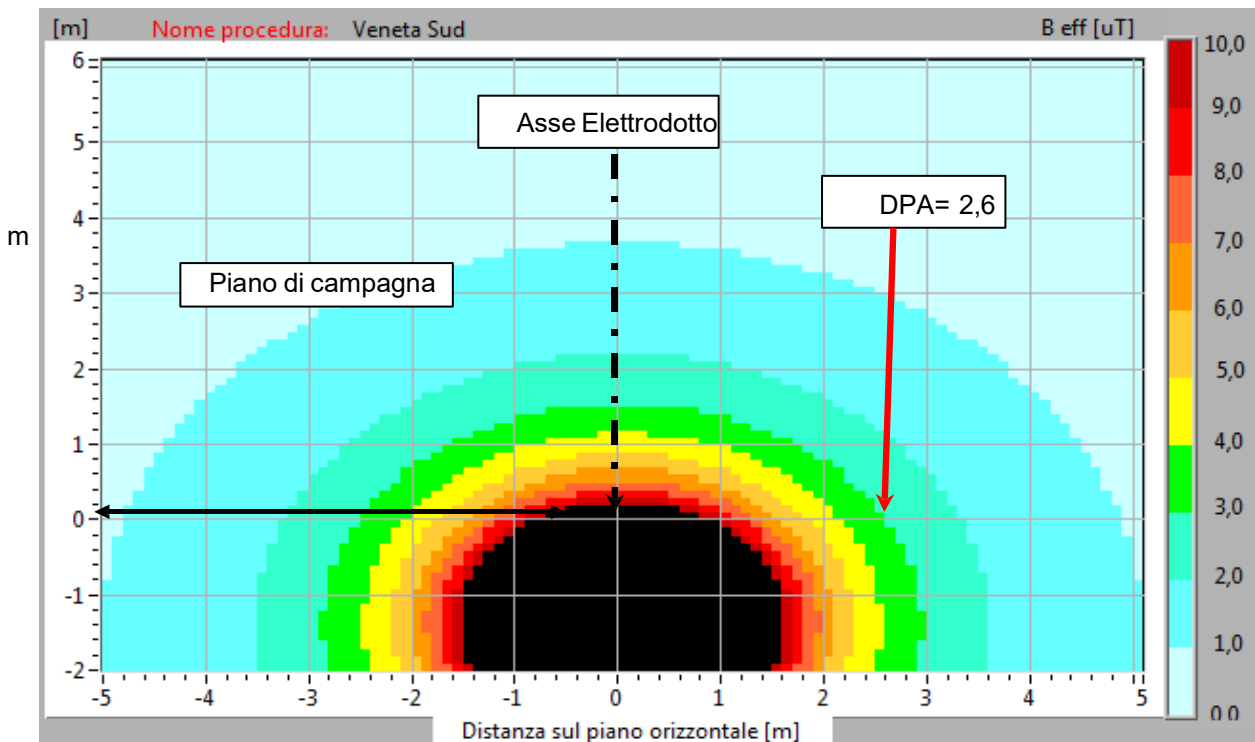
Figura 5 - Mappa verticale induzione magnetica (B) sezione tipo con indicazione della DPA - V=150\text{ kV} I=900\text{ A}
