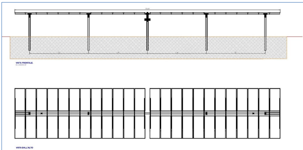
Vista frontale e vista dall'alto dei tracker con inclinazione 0°
