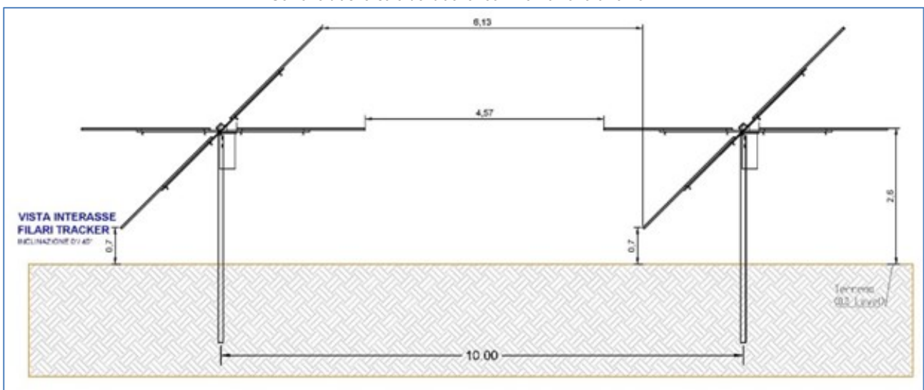
Figura 3.1. Prospetto trasversale e longitudinale delle strutture da installare
