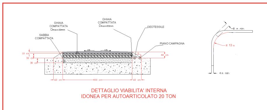
sezioni tipo
