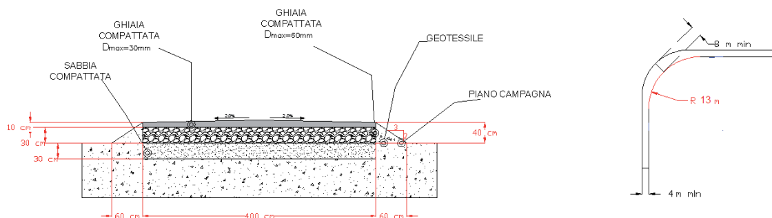
DETTAGLIO VIABILITA' INTERNA IDONEA PER AUTOARTICOLATO 20 TON
