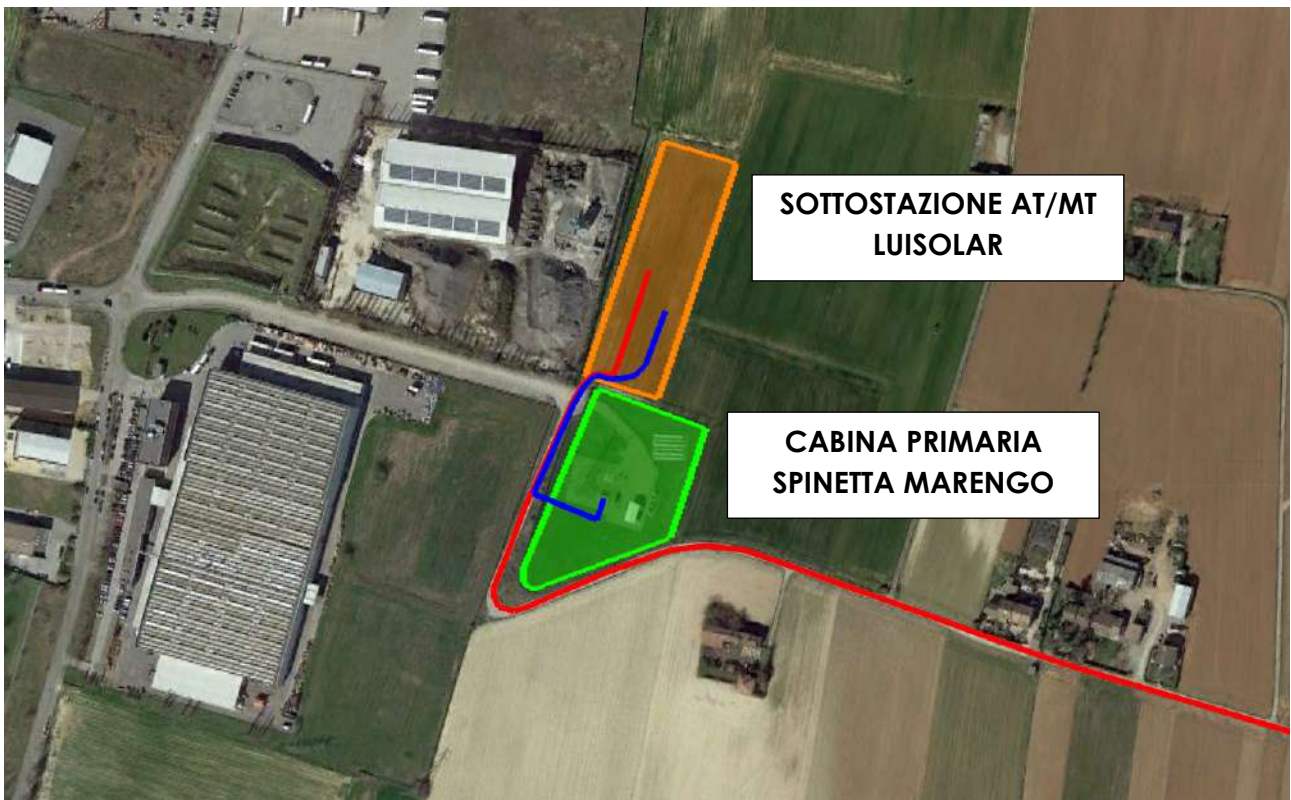
Dettaglio del tracciato del cavidotto AT
