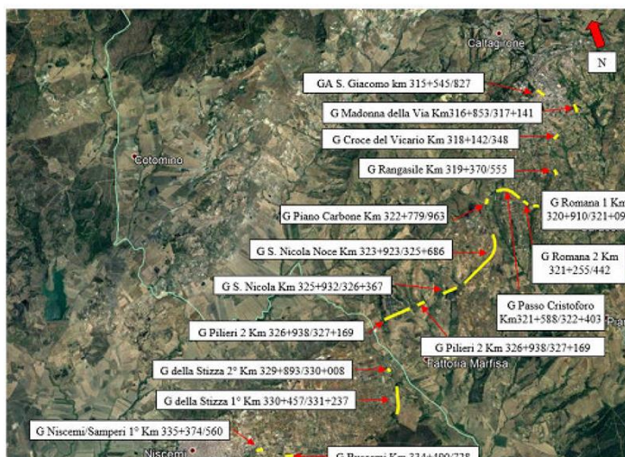
Figura 9: Gallerie presenti lungo il tracciato ferroviario del Lotto 1 Caltagirone-Niscemi
