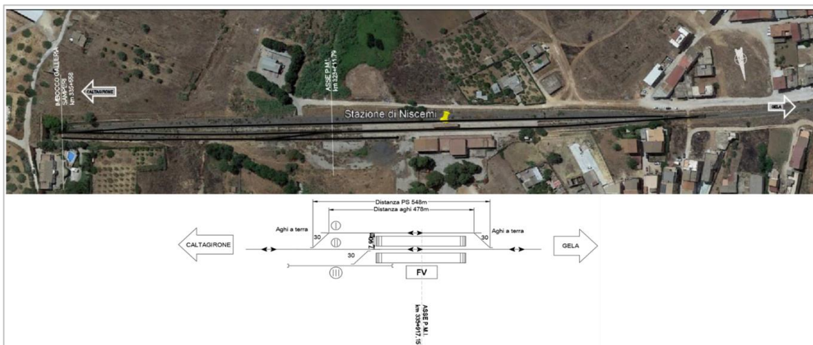
Figura 6: Stazione di Niscemi esistente
