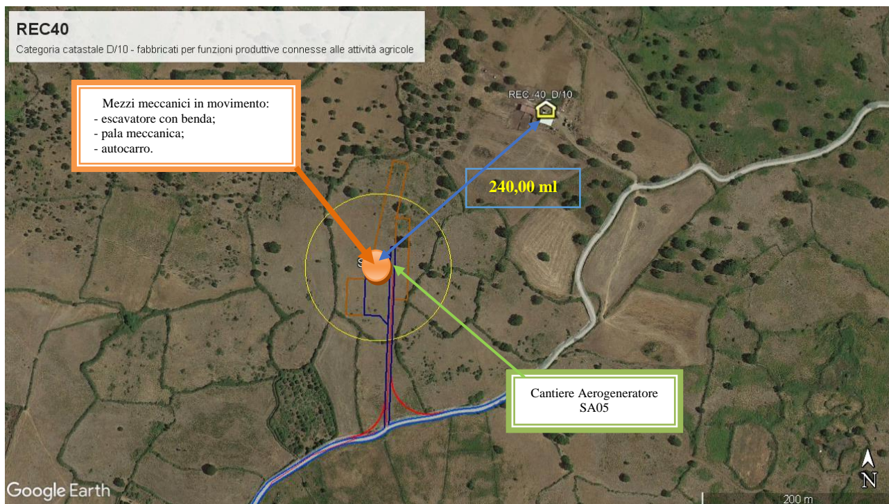
Figura 2: scenario 2 fondazioni WTG SA05
