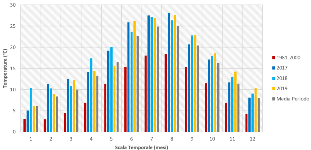
Figura 2.8: Distribuzione mensile della temperatura minima media nel periodo 2017 - 2019
