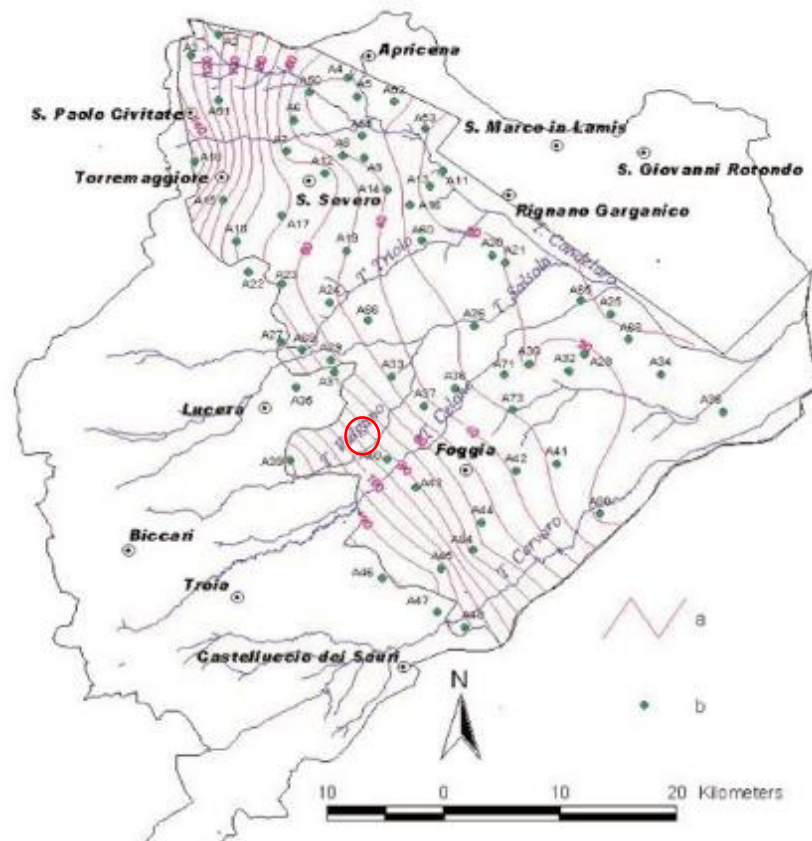
Figura 2.27: Ricostruzione della piezometria del 2002 (nel cerchio area in esame)
