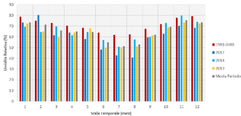
Figura 2.10: Distribuzione mensile dell'umidità relativa media nel periodo 2017 - 2019
