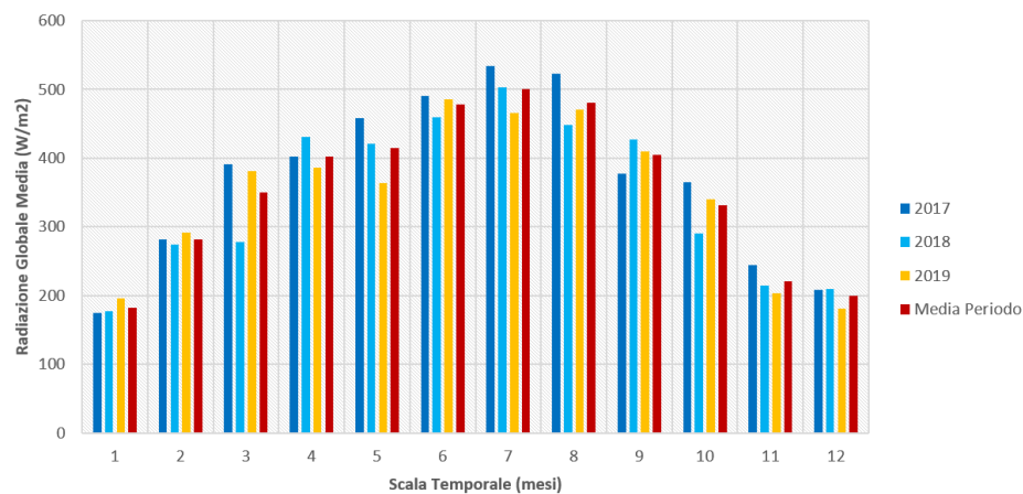
Figura 2.12: Distribuzione mensile della radiazione globale media 2017 - 2019
