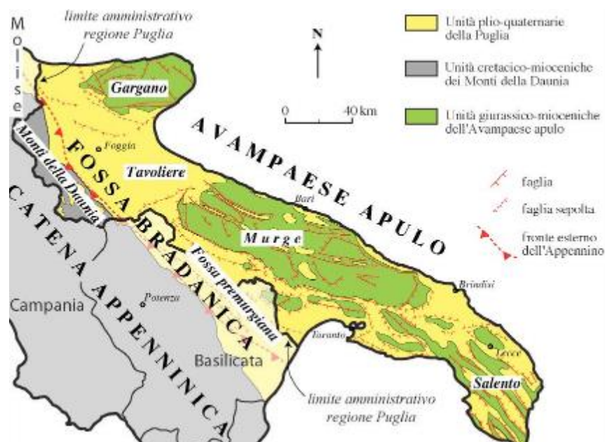
Figura 2.24: Carta geologica schematica della regione Puglia (da Pieri et alii, 1997, modificata)
