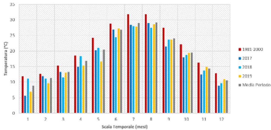
Figura 2.9: Distribuzione mensile della temperatura massima media nel periodo 2017 - 2019
