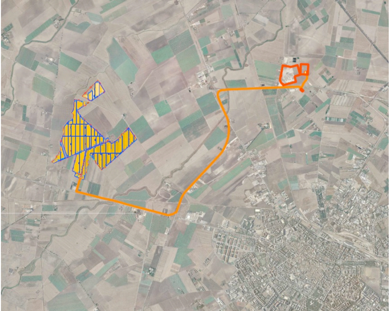
Figura 3.2: In arancio il percorso di connessione dal campo FV alla Sottostazione AT 380/150 kV Foggia
