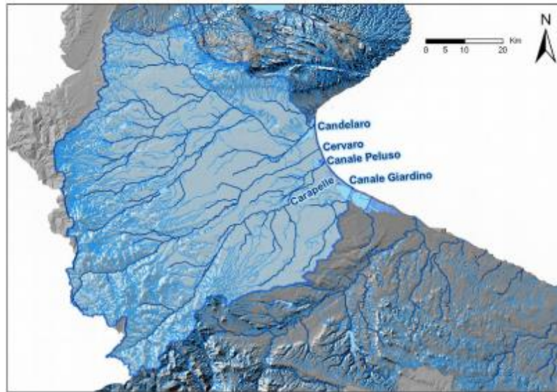
Figura 2.17: Corpi idrici superficiali (Relazione PGR - AdB Puglia)
