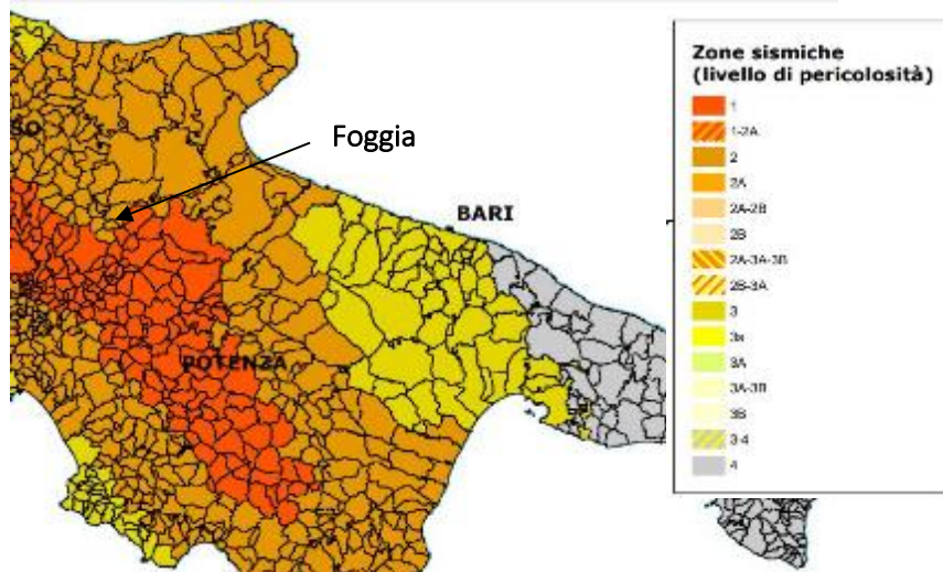
Figura 2.26: Classificazione sismica del gennaio 2019
