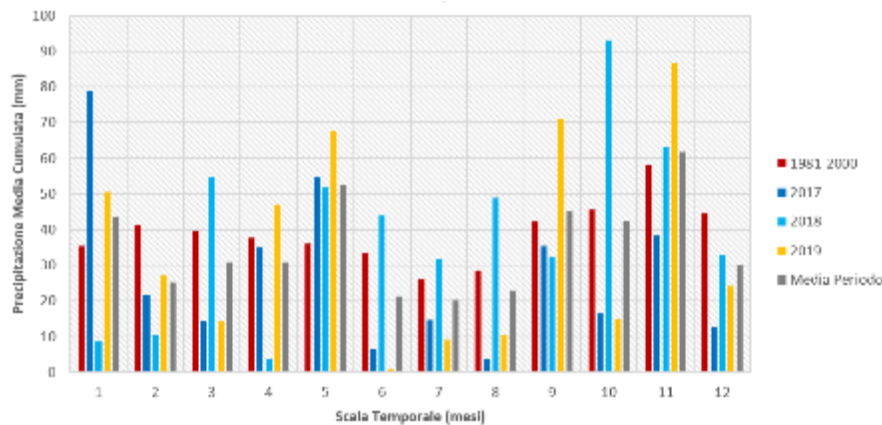
Figura 2.11: Distribuzione mensile delle precipitazioni medie cumulate 2017 - 2019
