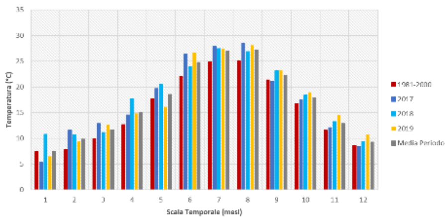
Figura 2.7: Distribuzione mensile della temperatura media nel periodo 2017 - 2019
