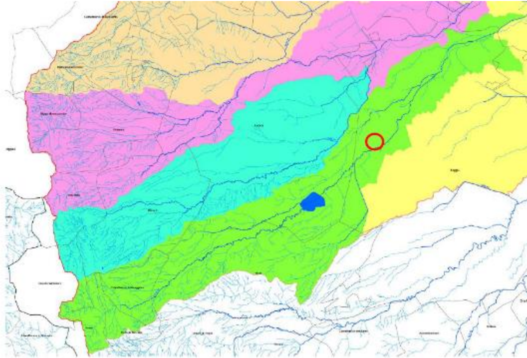
Figura 2.21: Stralcio cartografico Allegato 2.1 – “I Corsi d’acqua ricadenti nel bacino del Torrente Candelar con area contribuente uguale o maggiore di 25 kmq” – “Studio per la definizione delle opere necessarie alla messa in sicurezza del reticolo idraulico pugliese, con particolare riferimento alle aree del Gargano, delle coste ioniche e salentine della Regione Puglia” AdBP – Bacino Torrente Celone (CAND_03) in verde
