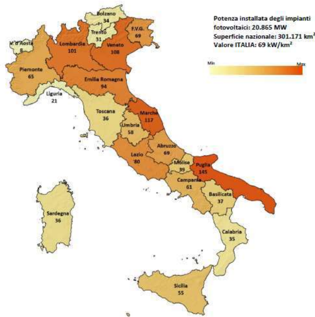
Figura 28 Densità della potenza installata a fine 2019 per regione (kW/km 2 )
