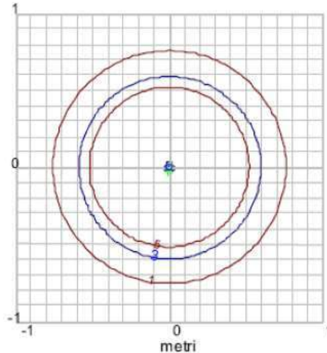
Figura Curve di equilivello per il campo magnetico di una linea MT in cavo elicordato interrata (dalla Norma CEI 106-11)
