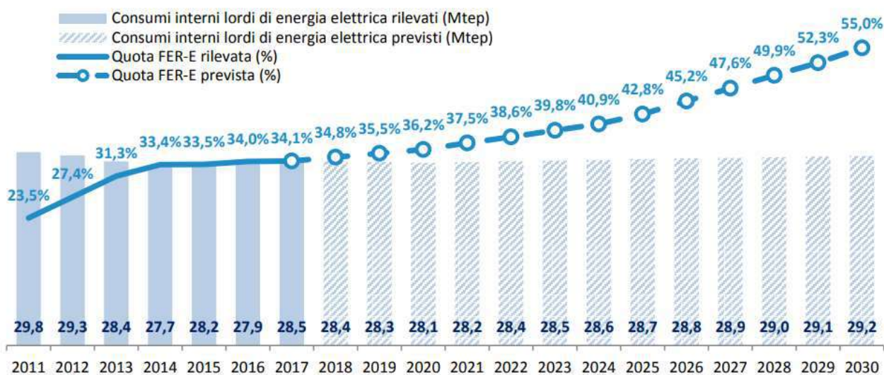
Figura 6 Traiettorie della quota FER elettrica [Fonte: GSE e RSE]
