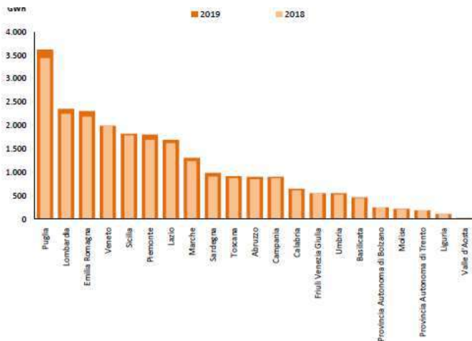
Figura 34 Produzione degli impianti fotovoltaici nelle regioni italiane nel 2018 e nel 2019
