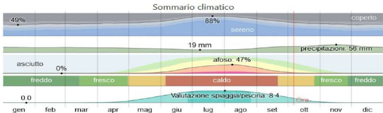
Figura 82 - Sommario climatico
