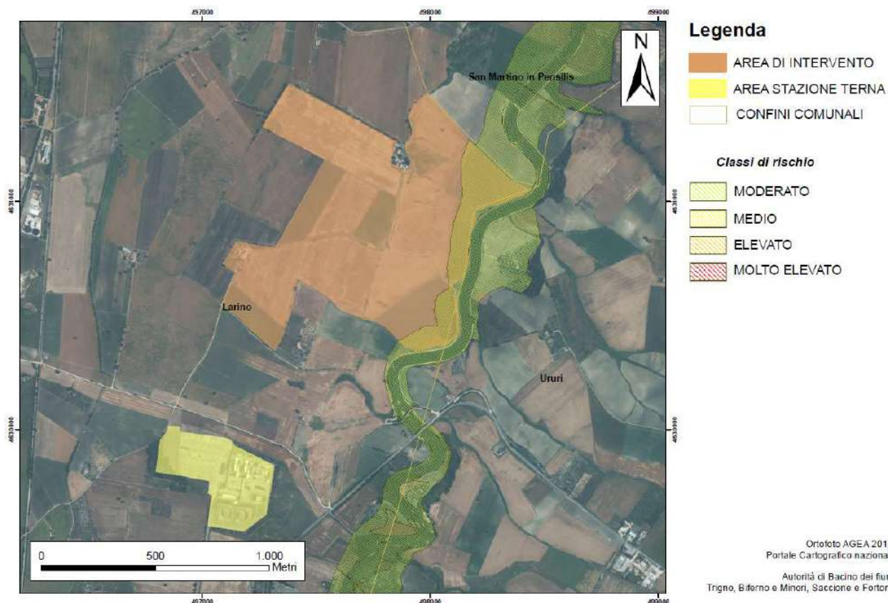
Figura 45 - Rischio idraulico
