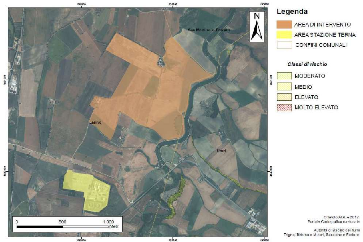
Figura 47 - Rischio frana
